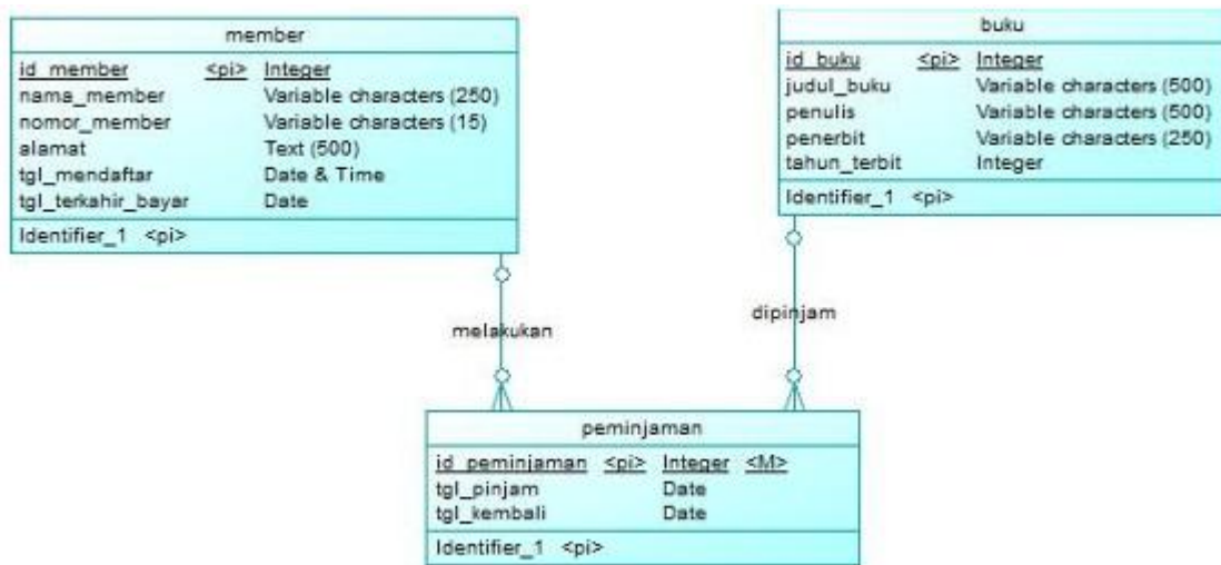
Gambar 1. Soal nomor 1
