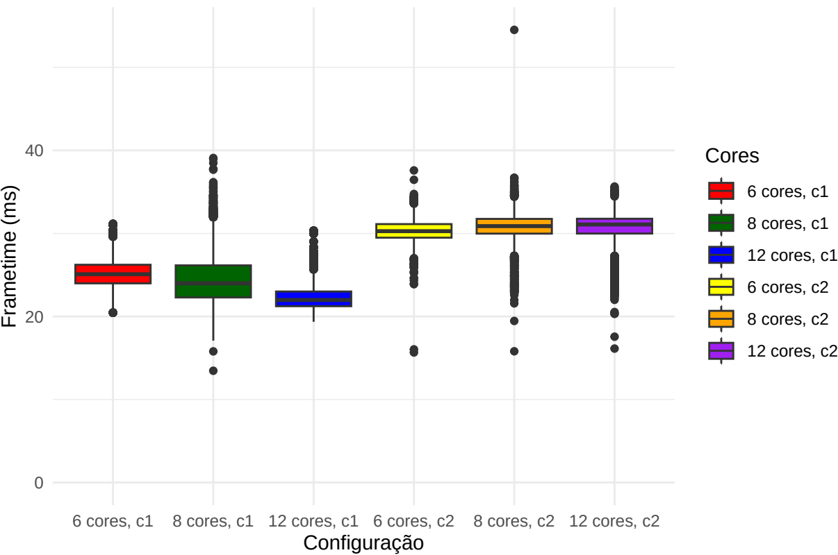
Variação de Frametime por número de cores – Ryzen 9 9900X
