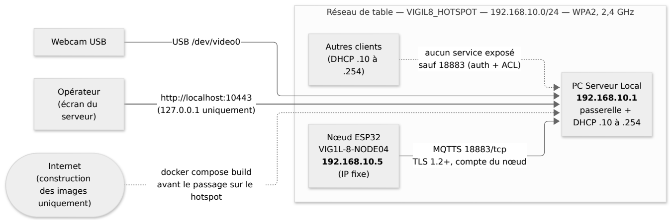
Figure 1 — Réseau de table : seul le port MQTT 18883 est exposé au réseau ; le dashboard n'écoute que sur la boucle locale du serveur.
