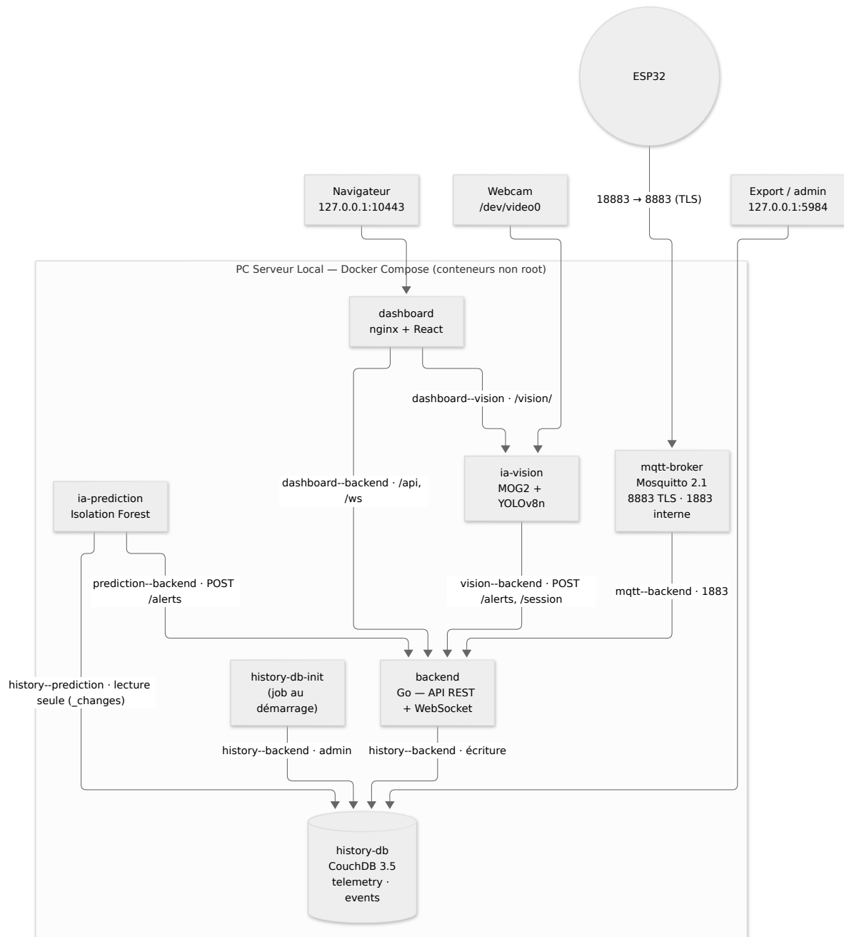
Figure 3 — Conteneurs, réseaux Docker et sens des échanges. Chaque réseau relie une paire de services.
