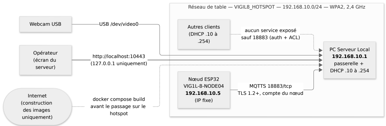
Figure 1 — Réseau de table : seul le port MQTTS 18883 est exposé au réseau ; le dashboard n'écoute que sur la boucle locale du serveur.
