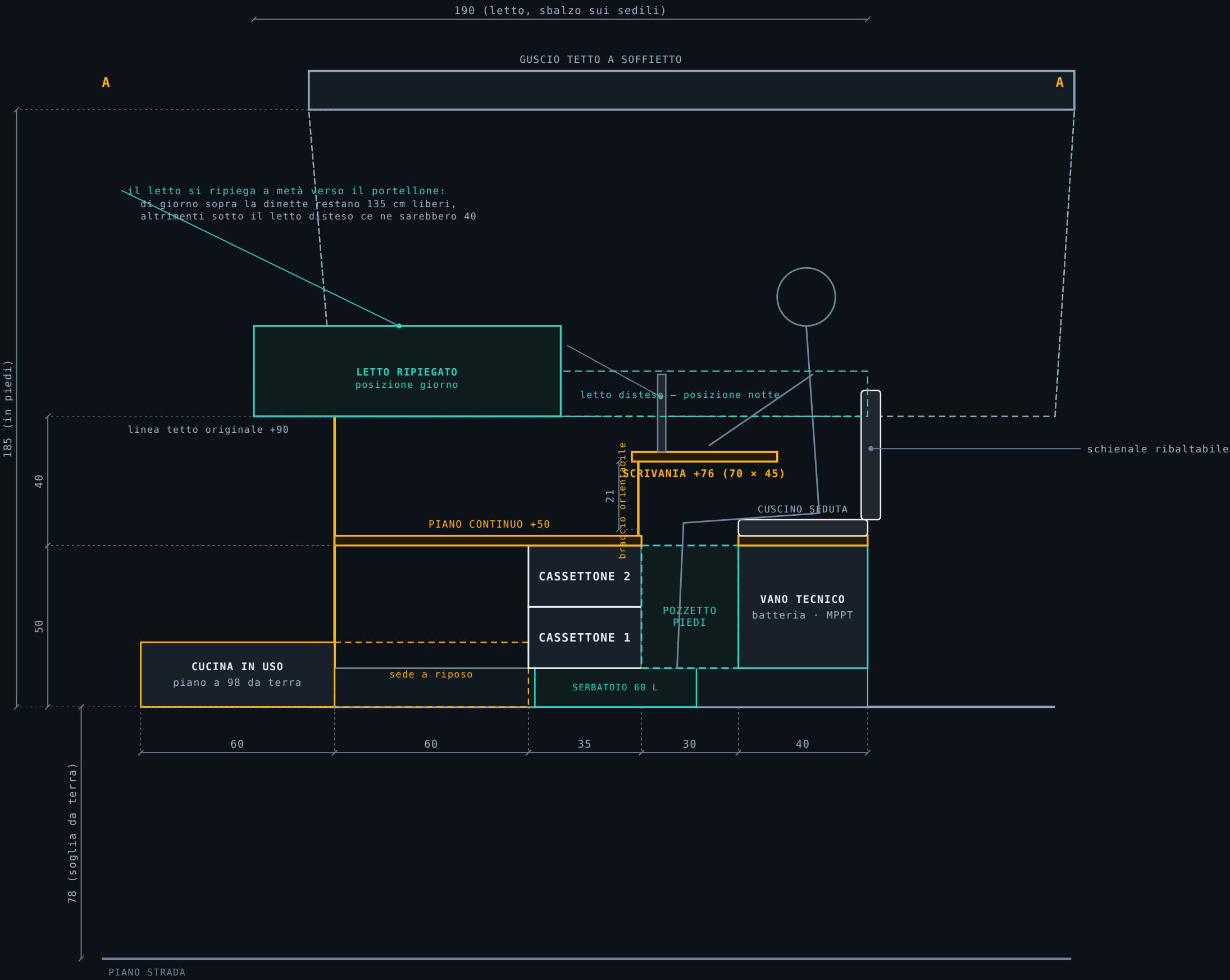
TAV. 2 – SEZIONE A-A
