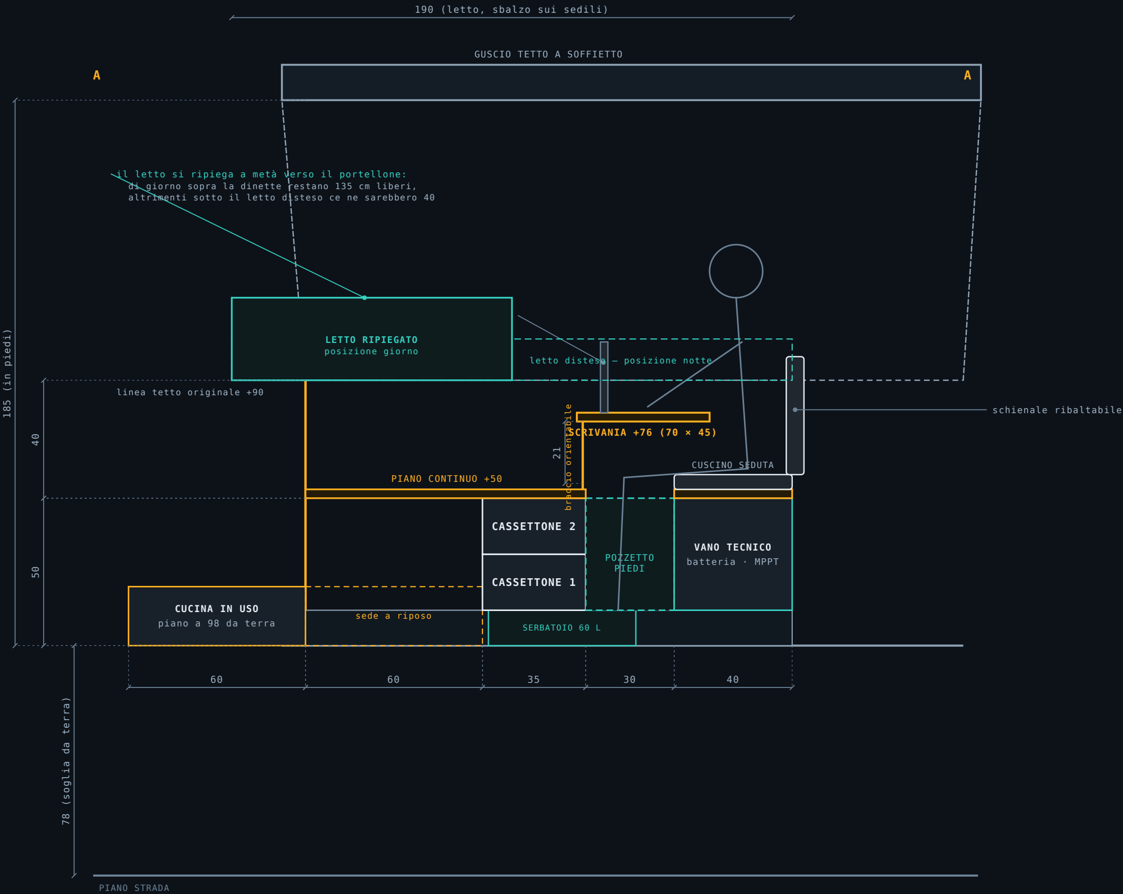
TAV. 2 – SEZIONE A-A
