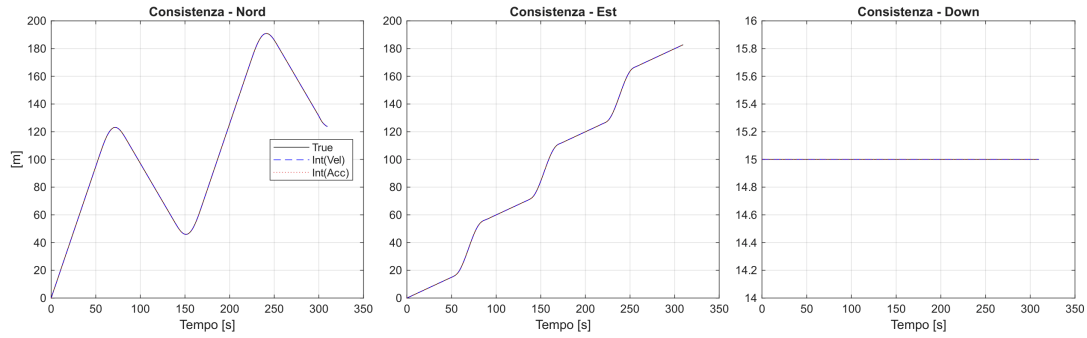
Figura 6.2: Verifica di consistenza dell'integrazione numerica sulle tre componenti spaziali.
