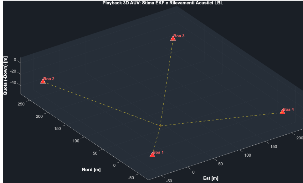
Figura 2.1: Disposizione spaziale delle 4 boe ( transponder ) rispetto all'area operativa sottomarina.
