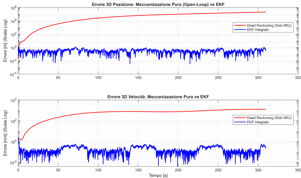
Figura 4.1: Norma dell'errore di posizione e velocità (scala logaritmica). Si nota la divergenza in anello aperto della meccanizzazione pura (rosso) contrapposta alla stabilità garantita dall'EKF (blu).
