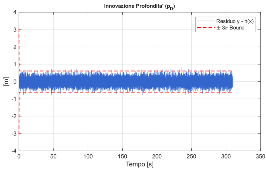
Figura 5.4: Innovazione della misura di profondità, con bound \pm 3\sigma .
