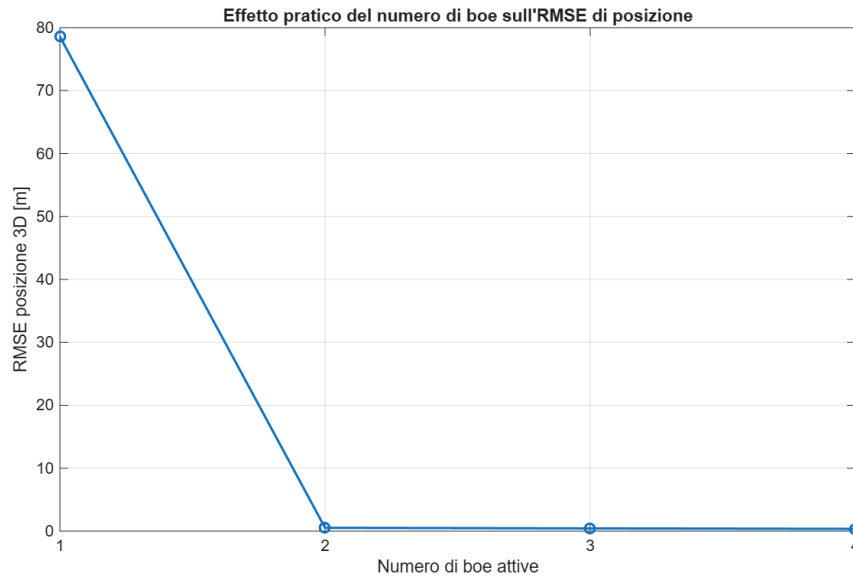
Figura 6.9: RMSE di posizione 3D al variare del numero di boe impiegate ( run_ablation.m ).
