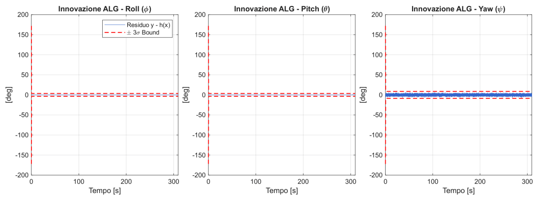
Figura 5.3: Innovazione delle pseudo-misure ALG (Roll, Pitch, Yaw), con bound \pm 3\sigma .
