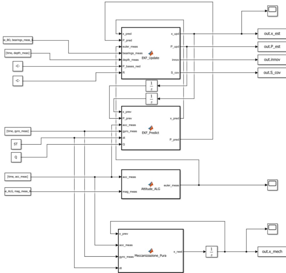
Figura 1.1: Architettura generale del sistema di navigazione in ambiente Simulink, comprensiva di sensoristica, meccanizzazione e stima EKF.
