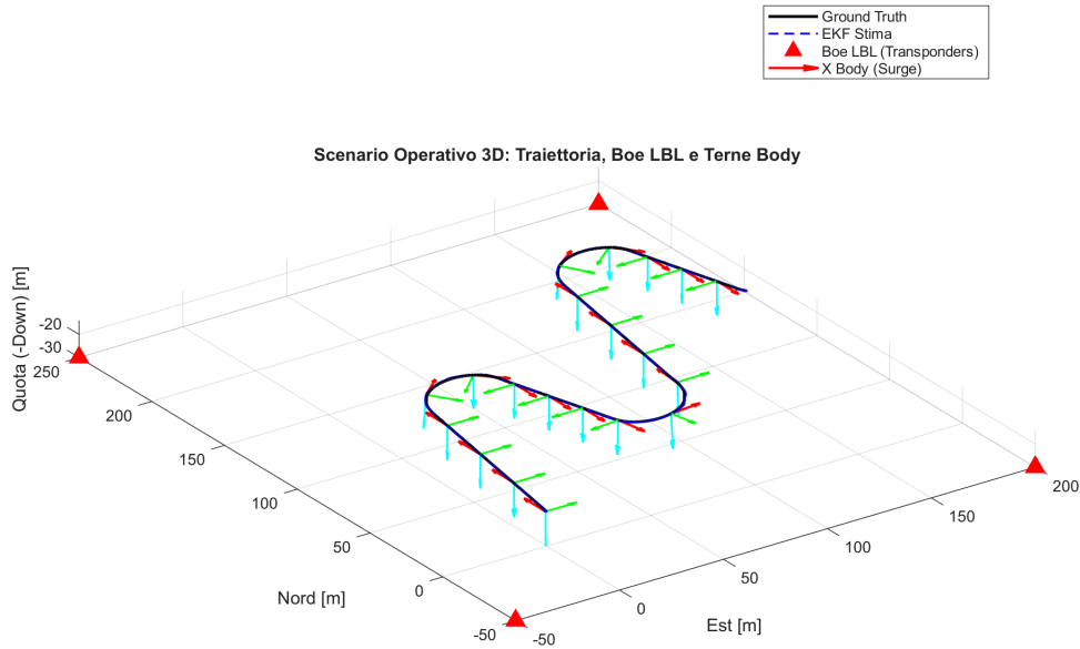
Figura 6.1: Playback 3D della missione con visualizzazione del sistema di riferimento locale (Assi Body ) e della rete di transponder acustici.
