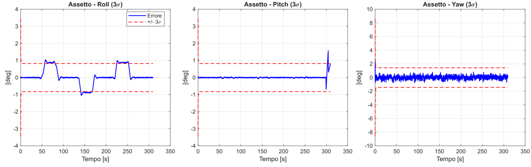
Figura 6.7: Errore di assetto EKF con intervalli di confidenza \pm 3\sigma .
