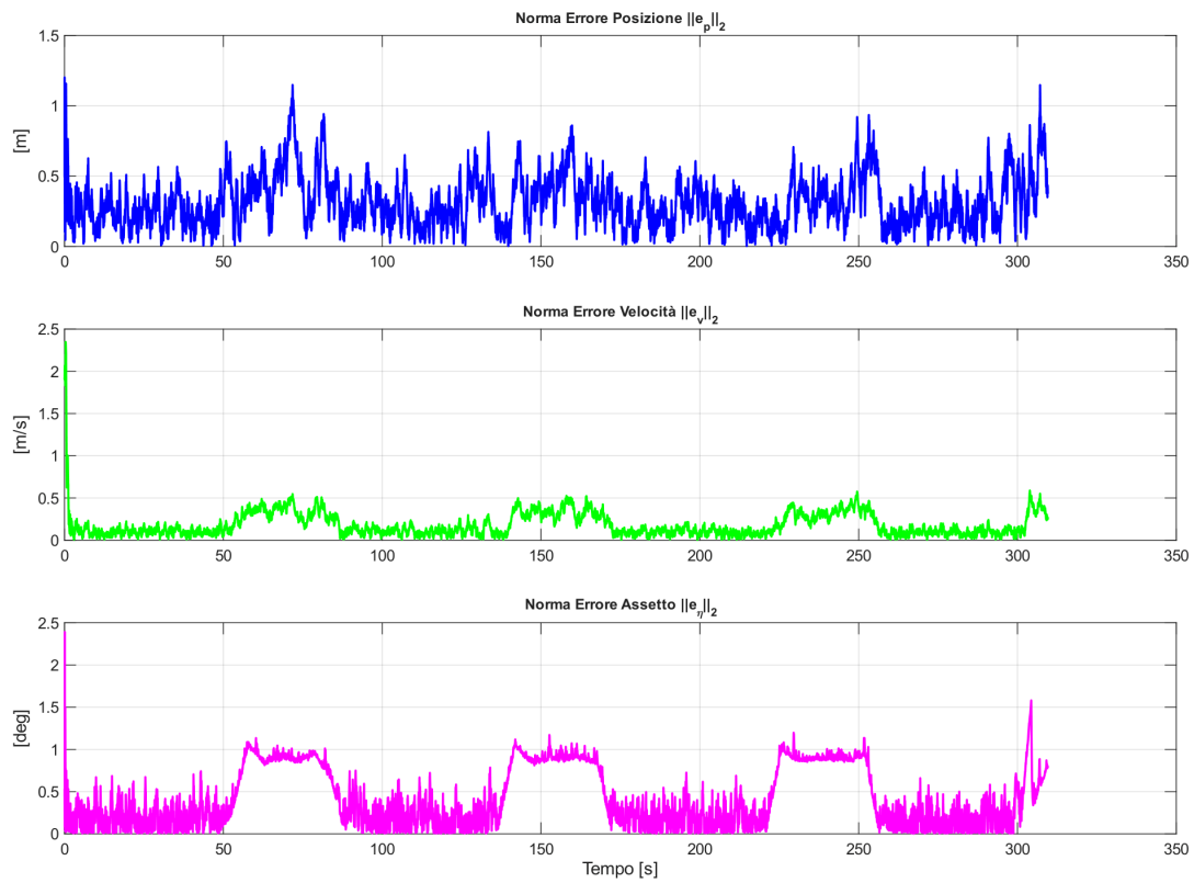
Figura 6.4: Norme euclidee degli errori di stima: posizione, velocità e assetto.
