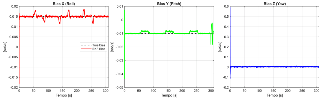
Figura 5.1: Dinamica di convergenza della stima EKF dei bias giroscopici (Roll, Pitch, Yaw) rispetto ai valori costanti reali di riferimento.
