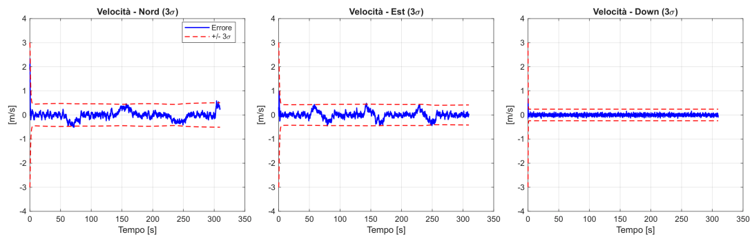
Figura 6.6: Errore di velocità EKF con intervalli di confidenza \pm 3\sigma .
