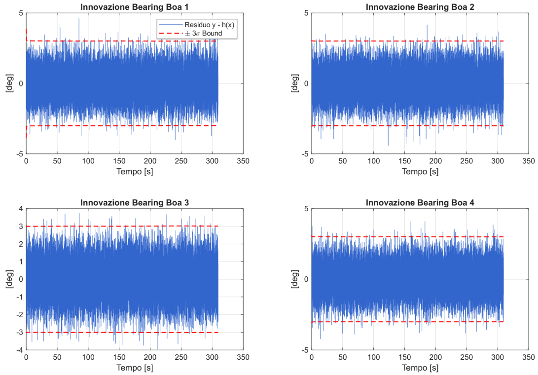
Figura 5.2: Innovazione angolare ( Bearing ) per le 4 boe. I residui si confrontano con i bound statistici \pm 3\sigma .
