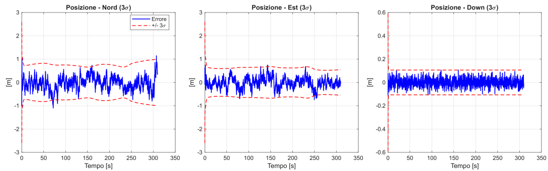
Figura 6.5: Errore di posizione EKF con intervalli di confidenza \pm 3\sigma .
