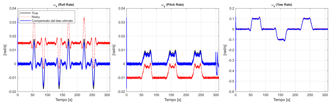
Figura 6.3: Dinamiche della velocità angolare in terna body : segnale ideale (True), misura grezza (Noisy), misura compensata dal bias stimato.
