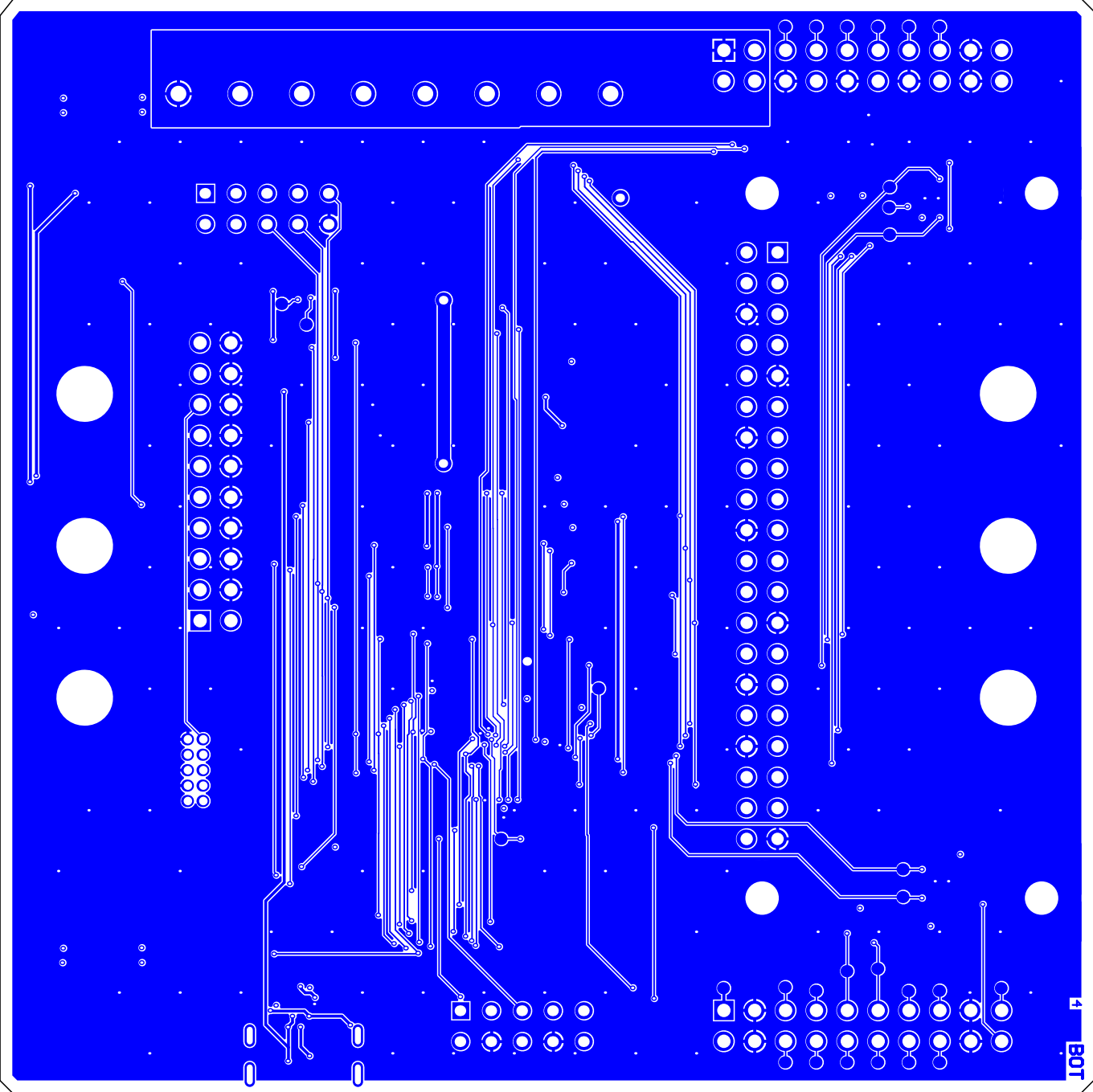
Bottom Layer (Scale 2:1)
