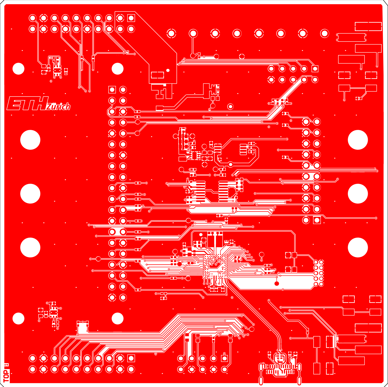
Top Layer (Scale 2:1)
