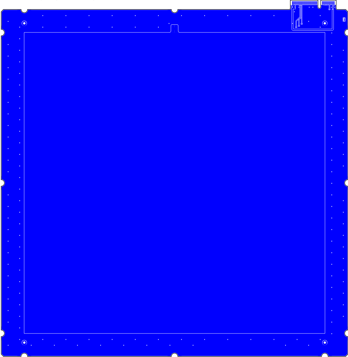
Bottom Layer (Scale 1:1)
