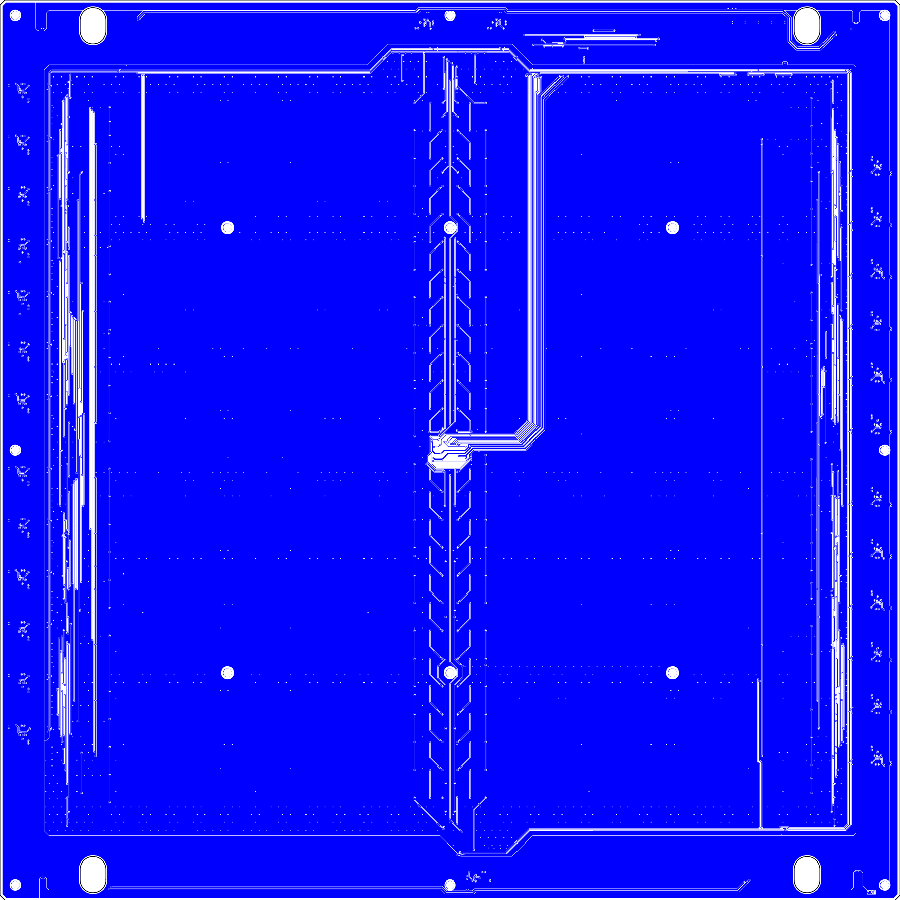
Bottom Layer (Scale 2:3)
