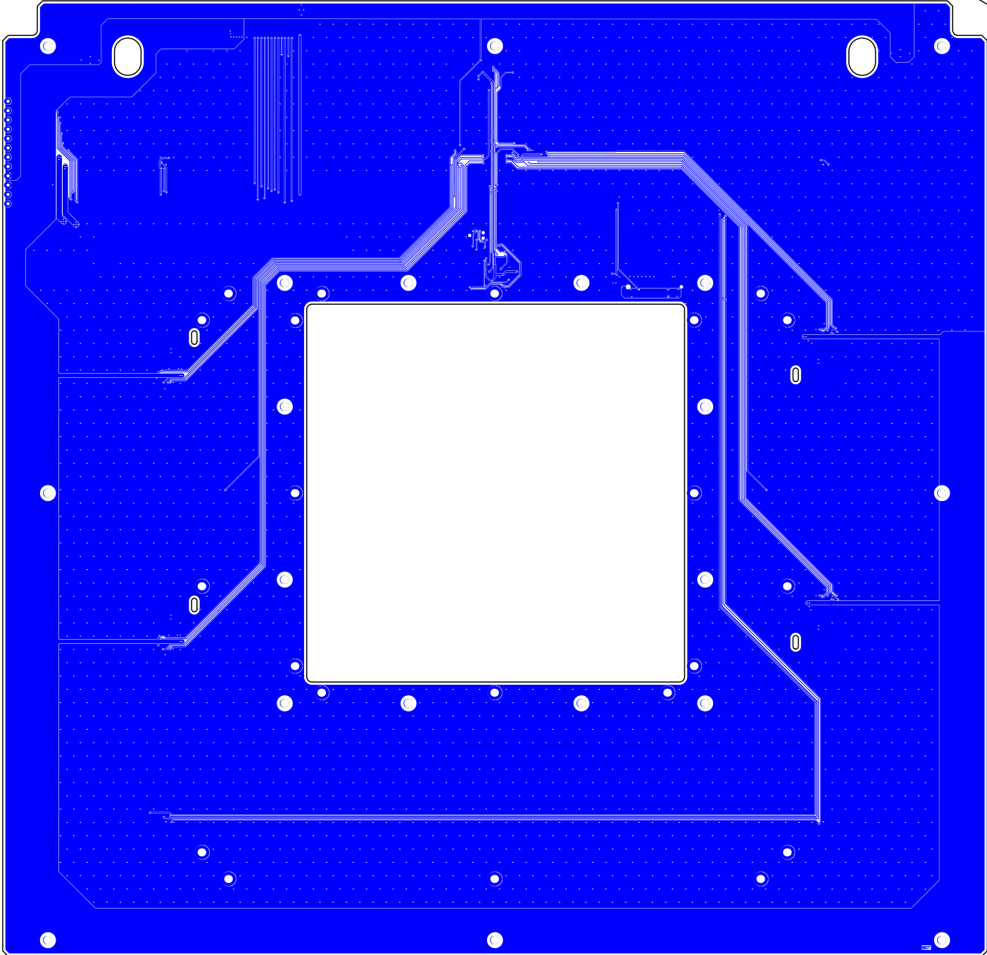
Bottom Layer (Scale 1:2)
