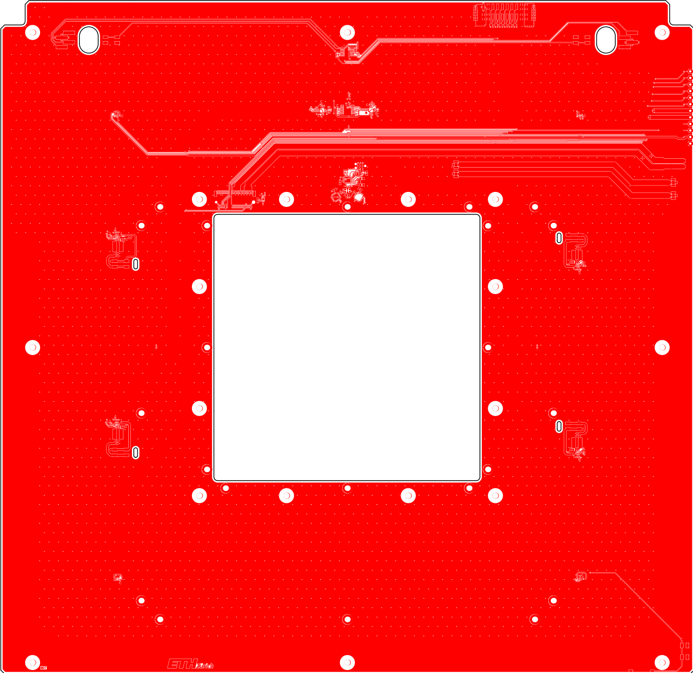
Top Layer (Scale 1:2)
