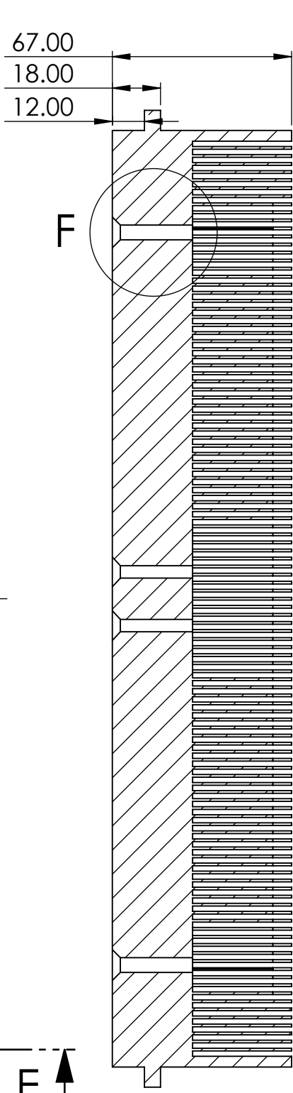
SECTION D-D SCALE 1 : 2
