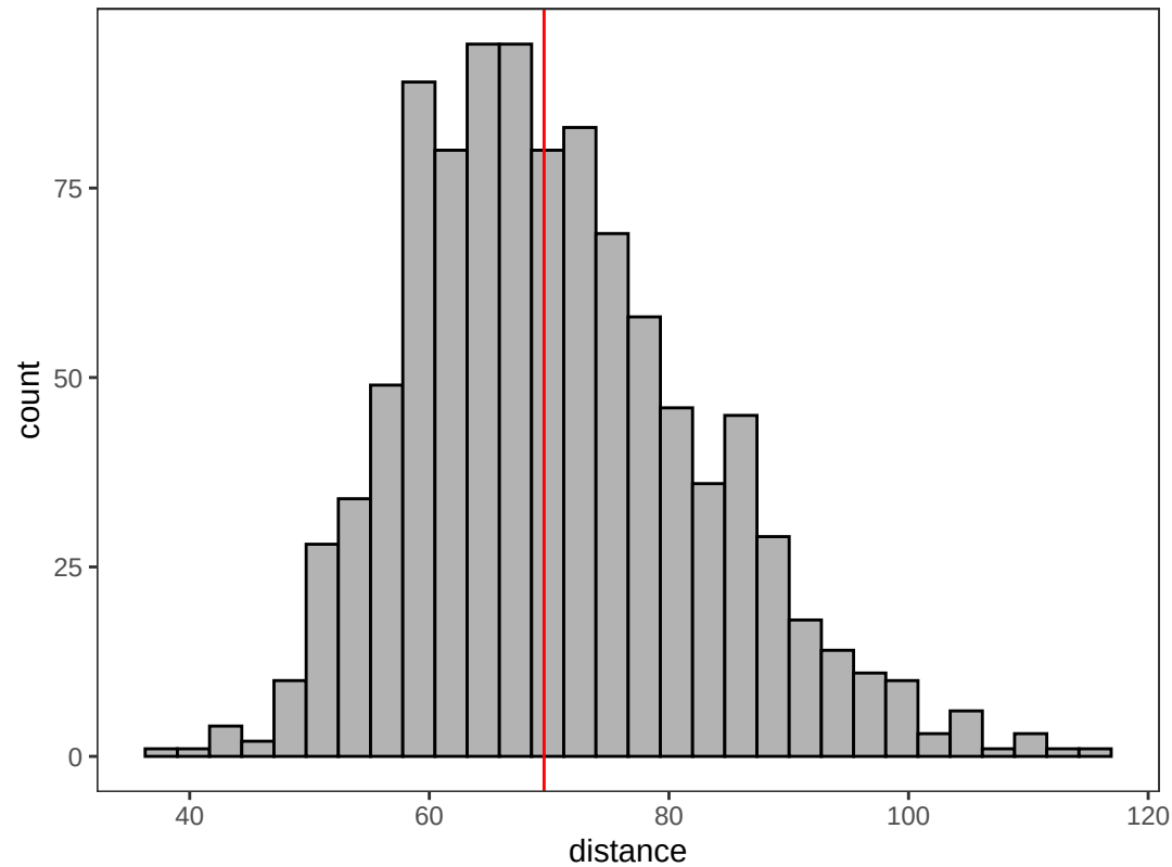
CTRL-vs-IFS kmeans.50
