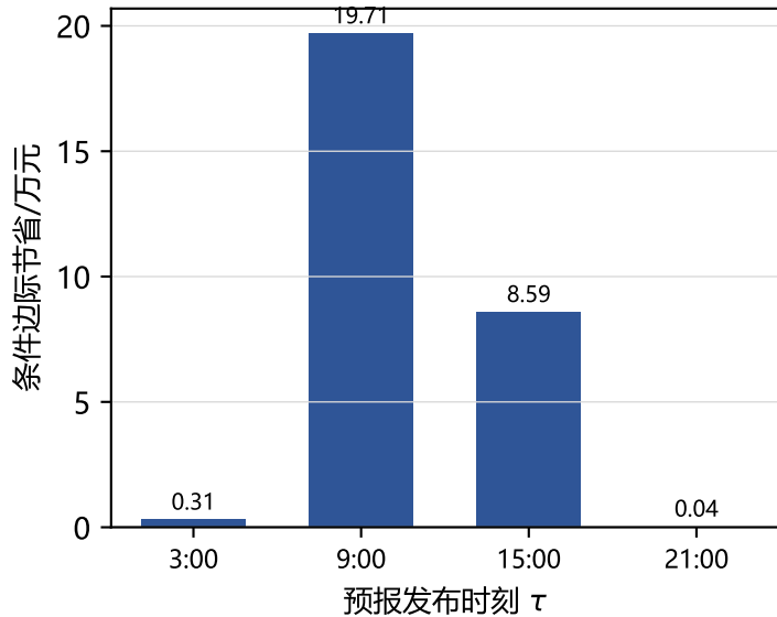
已有 6:00/12:00/18:00 预报时 新增一次完美光伏预报的条件价值
