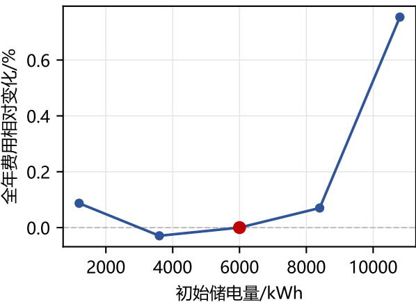
初始储电量
