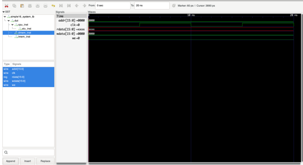
Şekil 7.4. Veri belleği (Data memory) modülüne ait adres, veri ve yazma kontrol sinyallerinin GTKWave üzerinde simülasyon dalga formu ile incelenmesi
