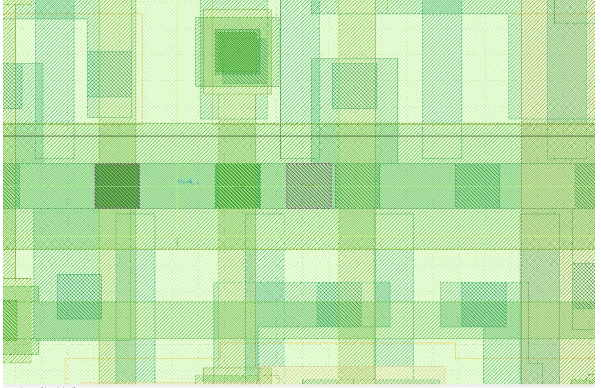
Şekil 5.14. Standart hücrelerin çekirdek alanı içerisindeki yerleşimi. %50 hedef doluluk oranı (PL_TARGET_DENSITY) hücreler arasında yeterli yönlendirme boşluğu bırakmıştır.
