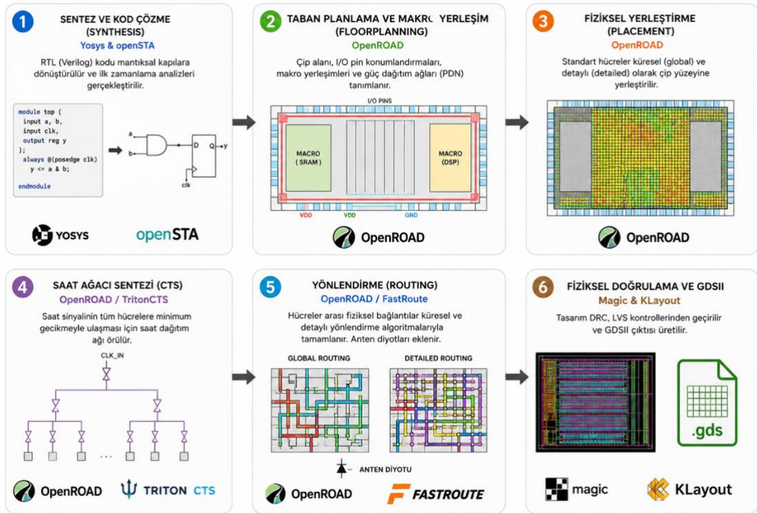
Şekil 1. OpenLane akışının temel katmanları
