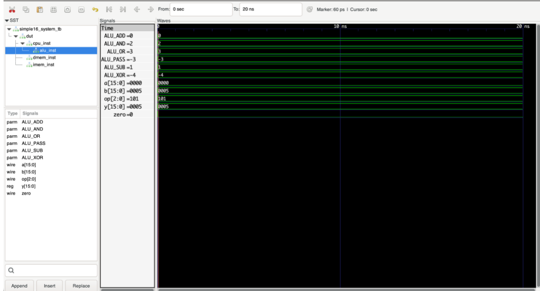
Şekil 7.3. ALU modülüne ait sinyallerin GTKWave üzerinde simülasyon dalga formu ile doğrulanması
