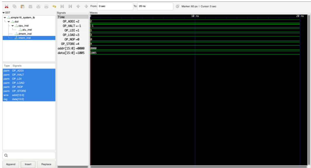
Şekil 7.5. Komut belleği (Instruction memory) modülüne ait opcode ve veri sinyallerinin GTKWave üzerinde simülasyon dalga formu ile doğrulanması
