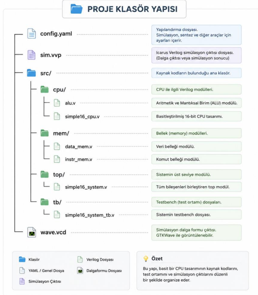
Şekil 4. Proje klasör yapısı
