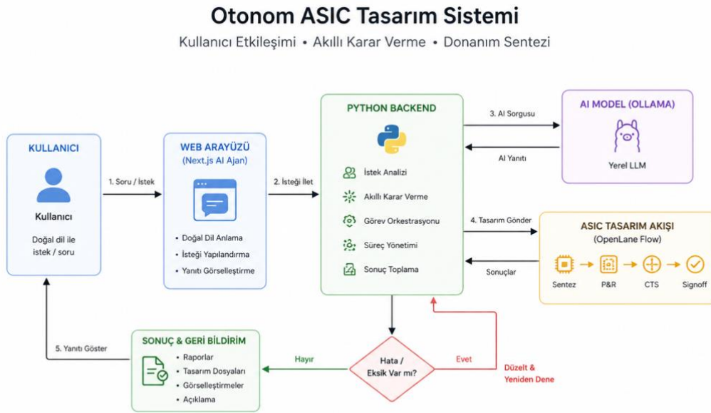
Şekil 2. Otonom ASIC tasarım sistemi
