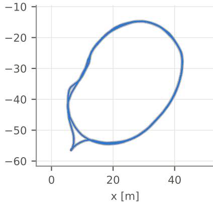
Newer College quad_easy (Ouster 128) APE: KISS-SLAM 0.10 m · ours 0.08 m
