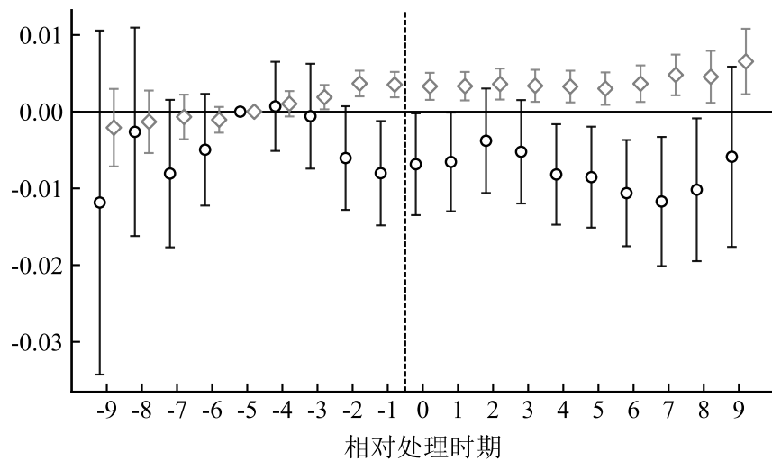
(c) SA
