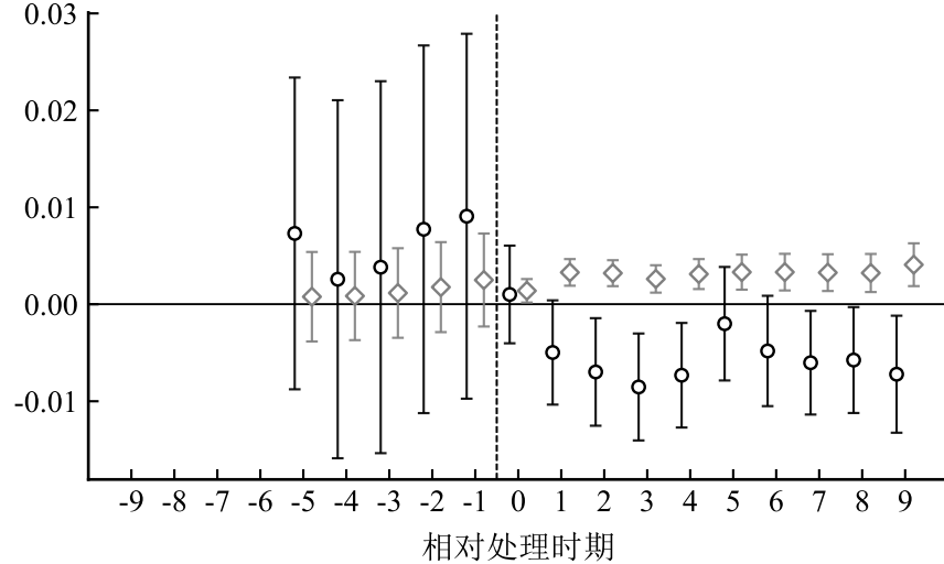
(d) BJS
