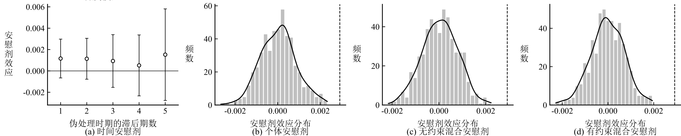
Panel B: 研发投入 (R&D)
