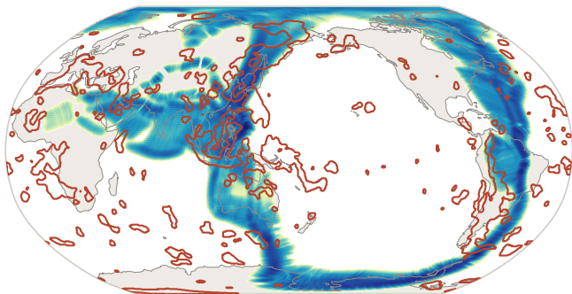
c 100–200 Ma
