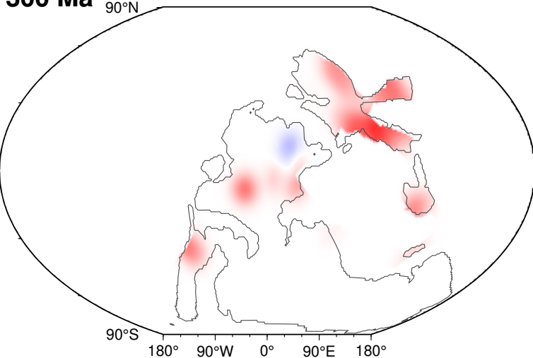
300 Ma delta z
