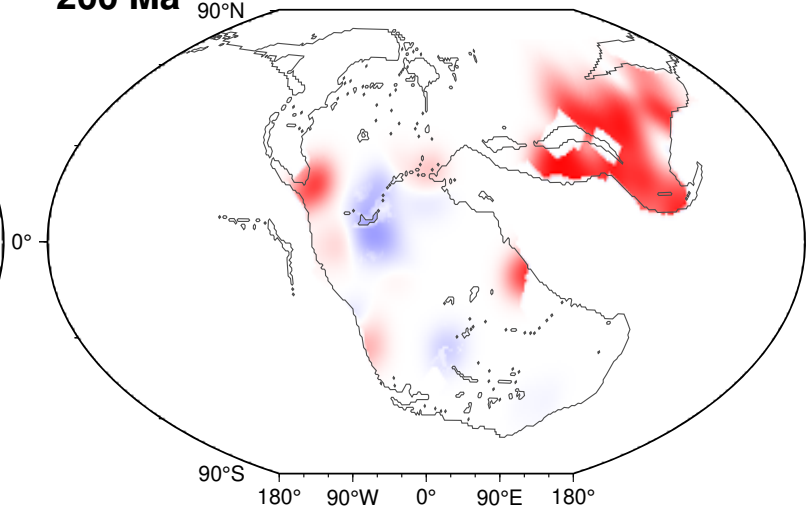
200 Ma delta z
