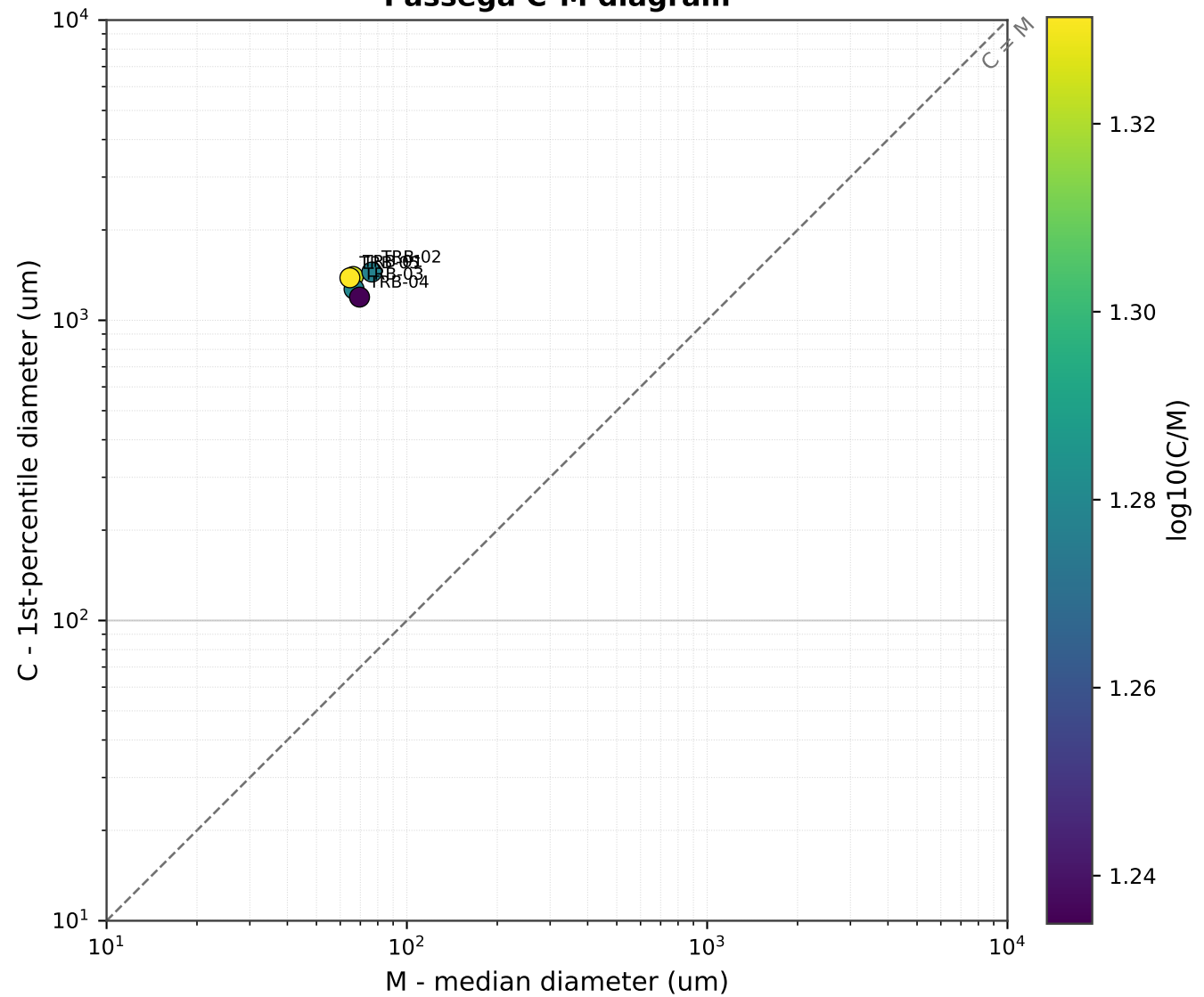
Passega C-M diagram
