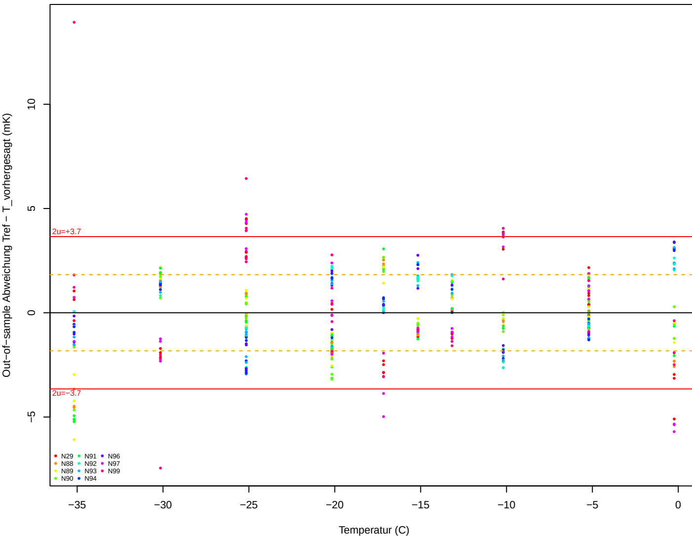
Kalibrierte NTCs: out-of-sample Abweichungen (Leave-one-T-out CV)
