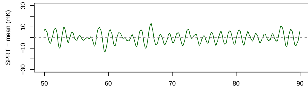
R2 SP -25 C (ok=FALSE) | sd 4.8 mK
