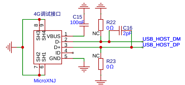
4G模块USB接口
