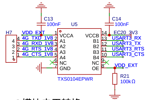
4G模块电平转换
