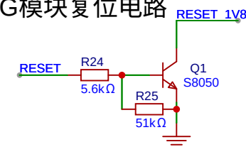
4G模块复位电路
