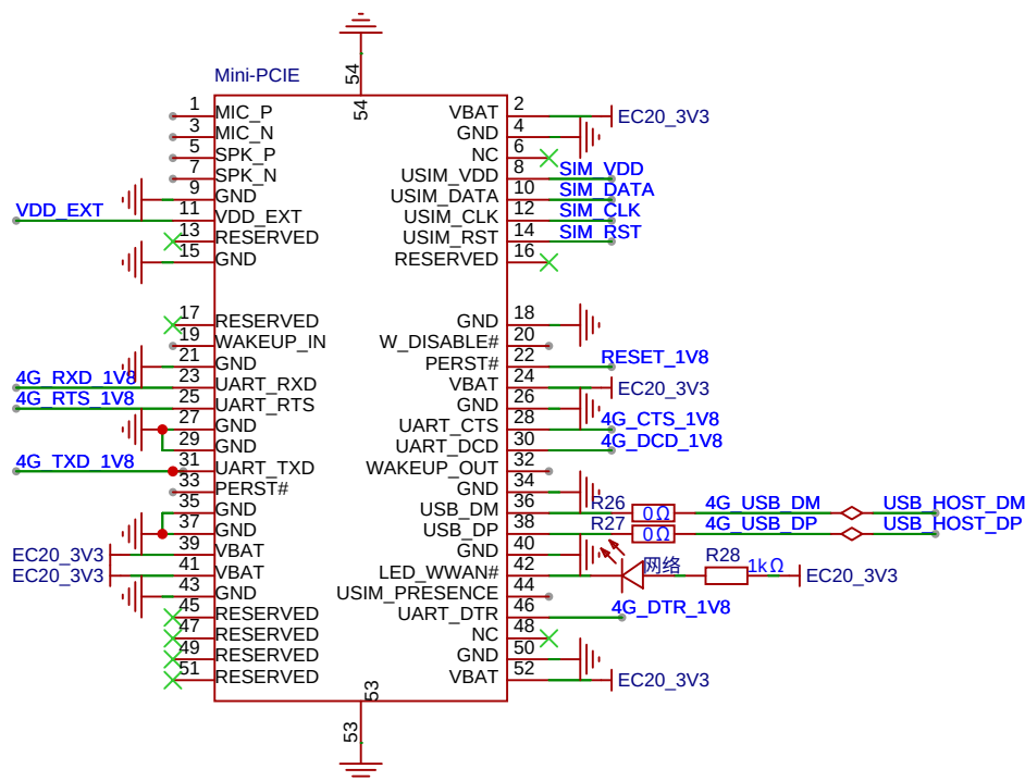
EC20 MINI-PCIE模块
