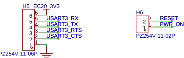
EC20 MINI-PCIE模块
