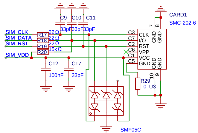
SIM卡电路
