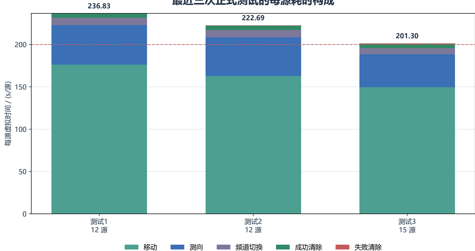
最近三次正式测试的每源耗时构成
