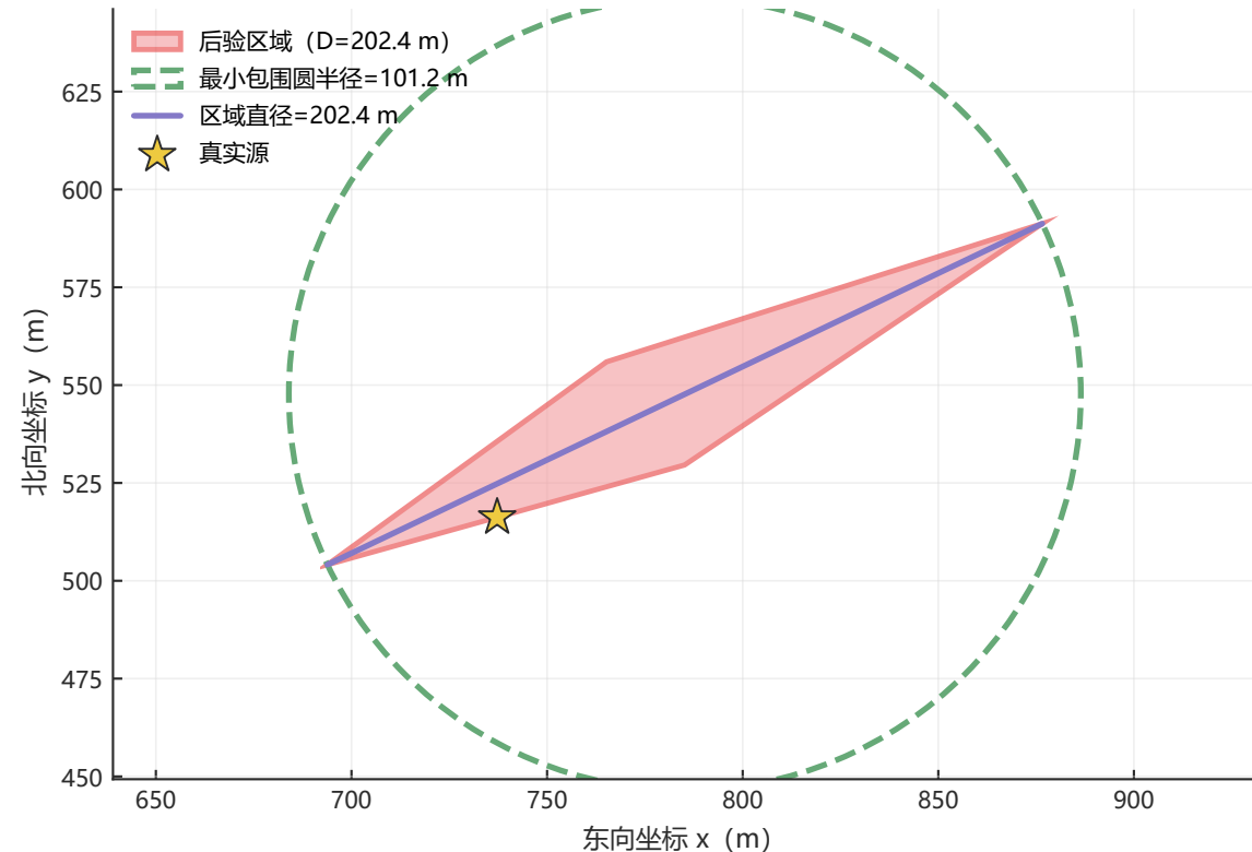
第二次观测后 (测试误差=+1.0°)
