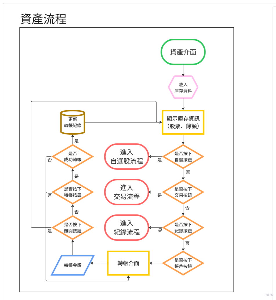
Figure 5: 資產庫存與轉帳流程圖
