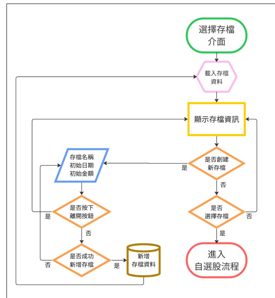
Figure 2: 選擇與建立存檔流程圖
