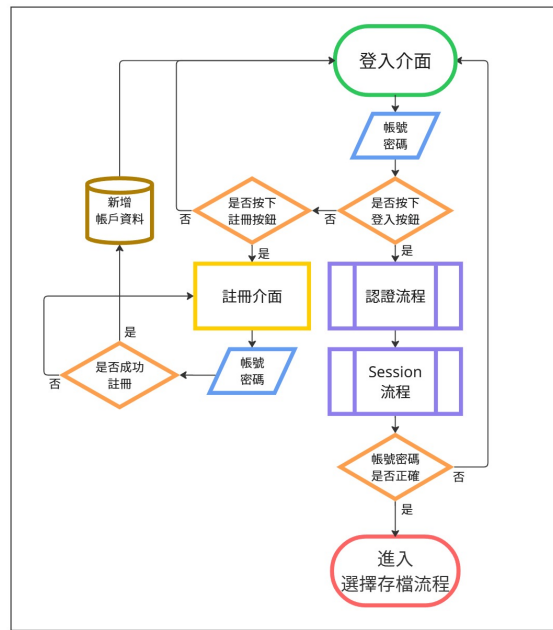
Figure 1: 登入與註冊流程圖
