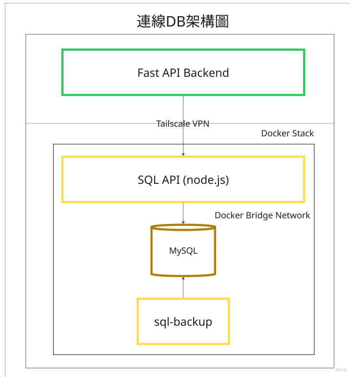
Figure 23: 資料庫存取架構圖
