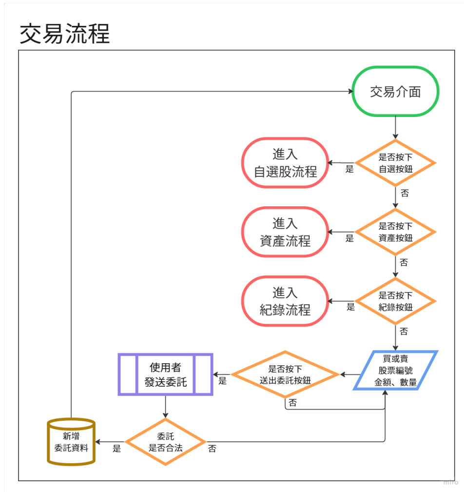
Figure 4: 交易下單流程圖
