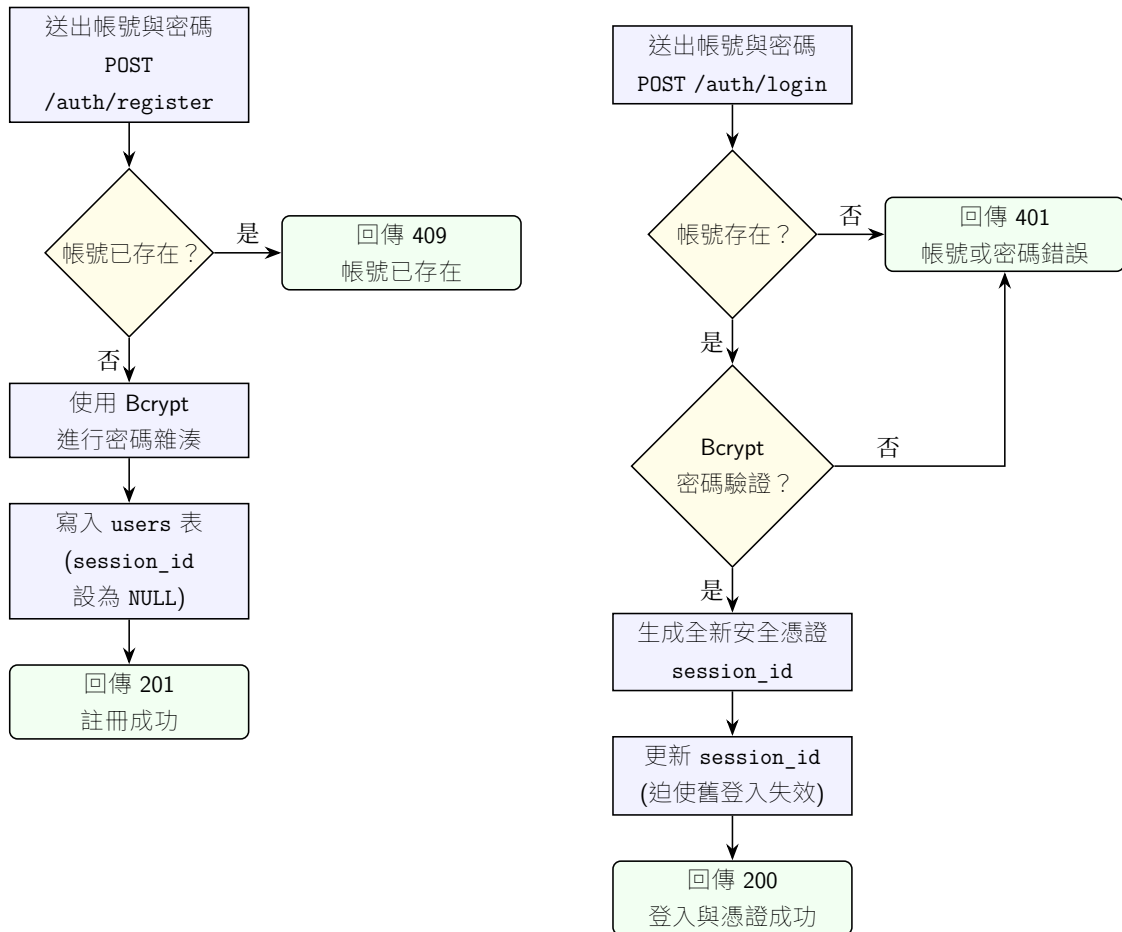
Figure 8: 後端身分驗證（註冊與登入）流程圖
