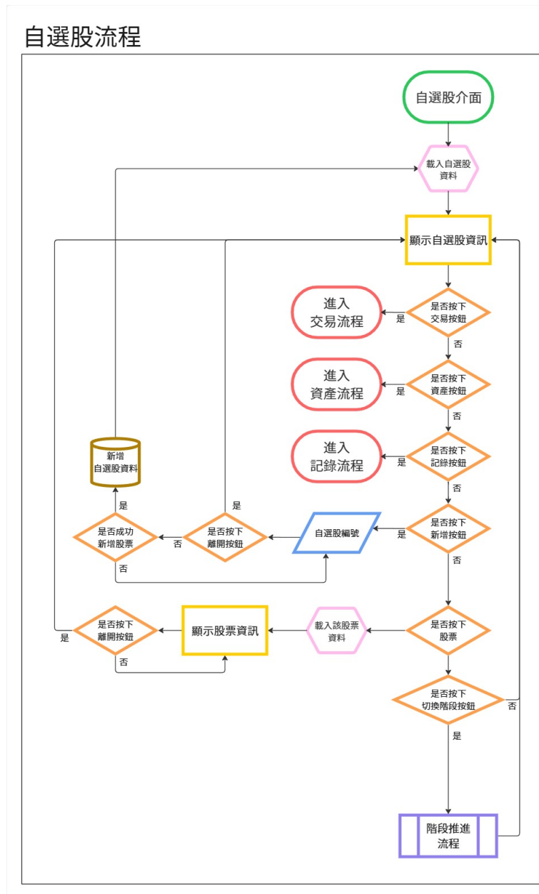
Figure 3: 自選股主頁面流程圖
