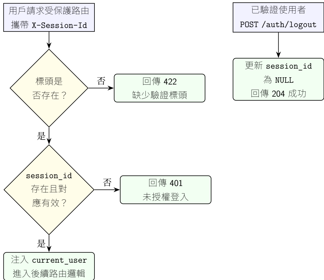
Figure 9: 受保護 API 請求驗證與登出流程圖
