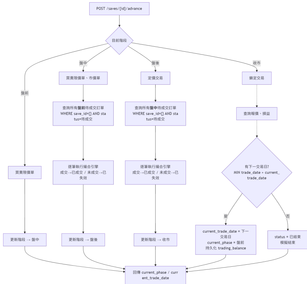
Figure 10: 階段推進邏輯圖
