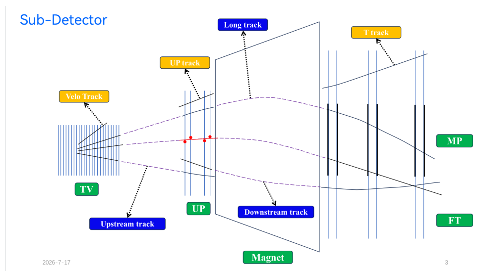
图 1: LHCb 升级二期子探测器布局示意图。TV (Vertex Tracker) 位于对撞点附近，UP (Upstream Tracker) 和磁铁位于中游，MT (Main Tracker, 分为 MP 和 FT) 位于下游。紫色虚线表示粒子径迹，红色圆点表示探测器击中。图中展示了 Velo track、Upstream track、Long track、Downstream track 和 T track 等不同类型径迹的分类。
