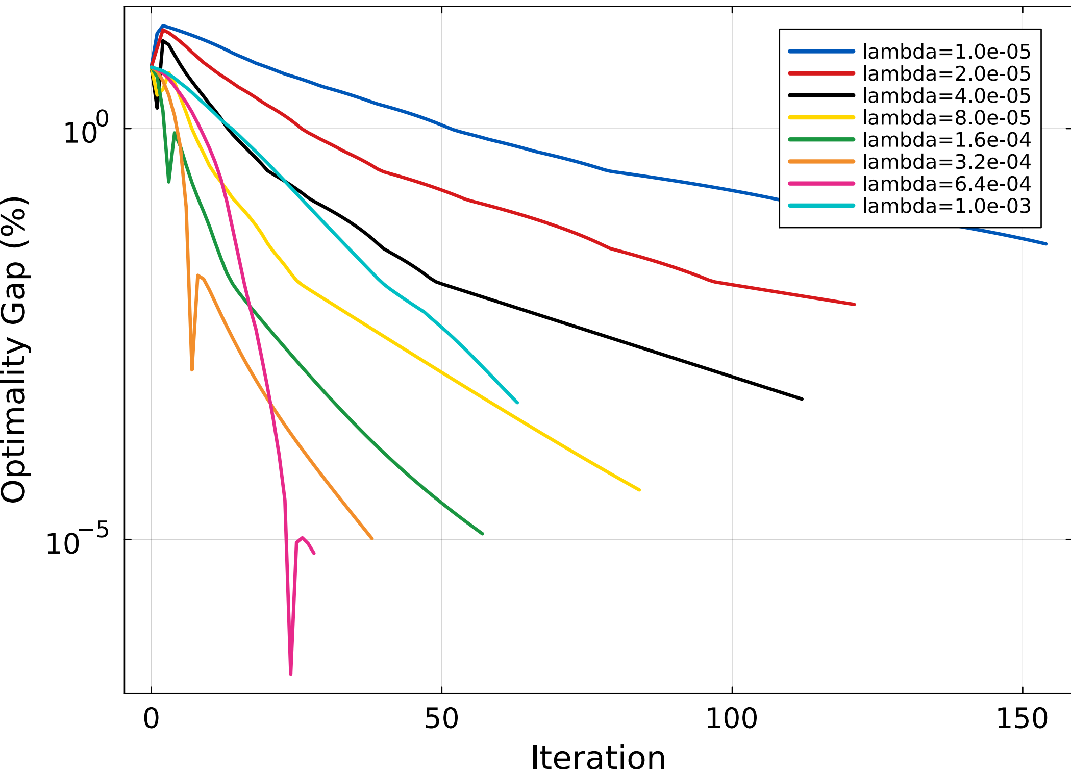
fADMM
