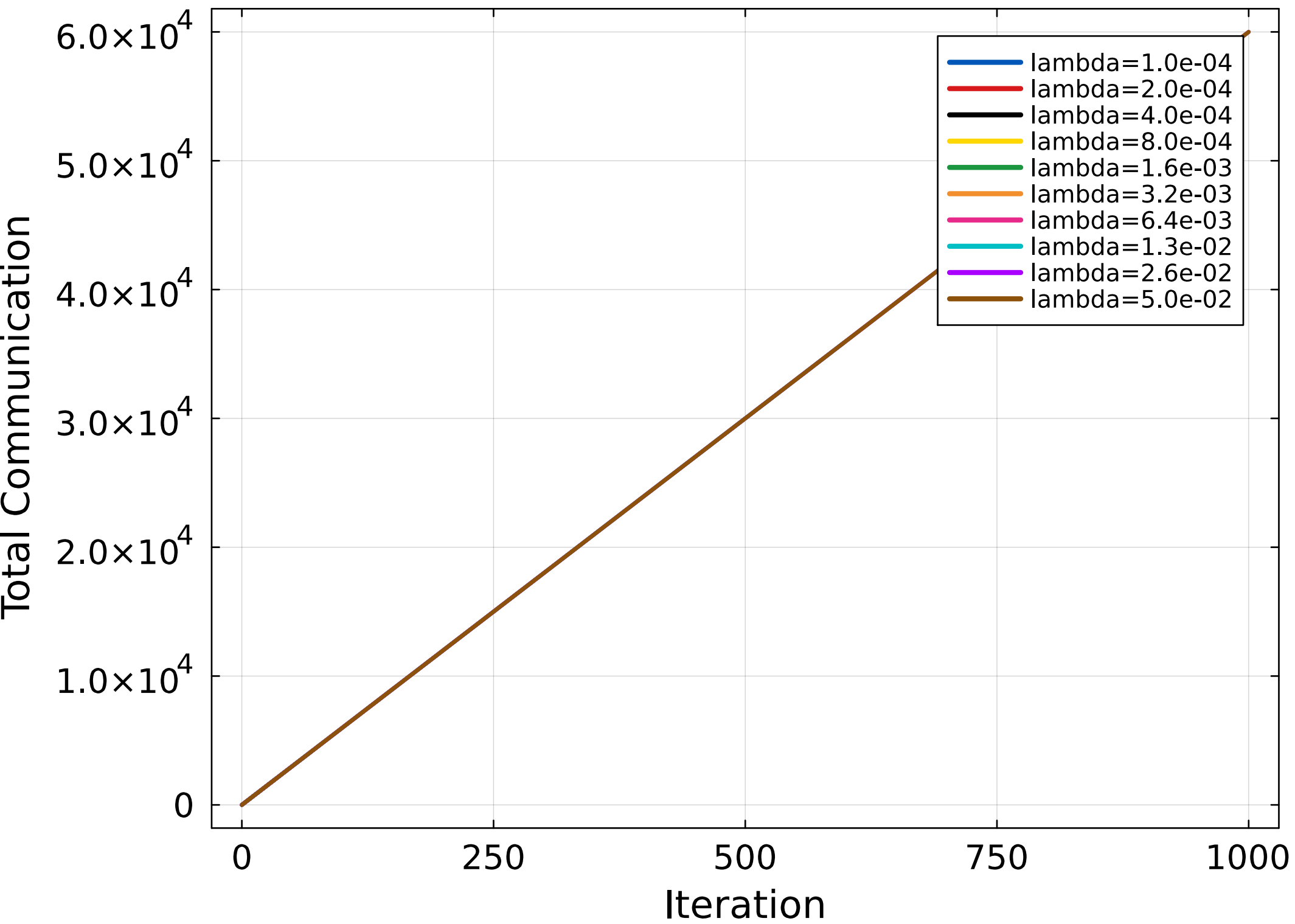
hADMM
