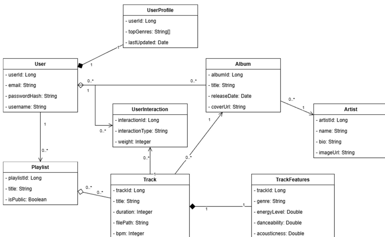
Рисунок 3.3 – Диаграмма классов
