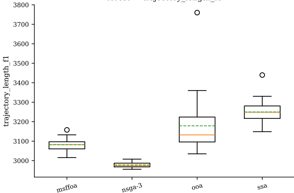
forest — trajectory_length_f1
