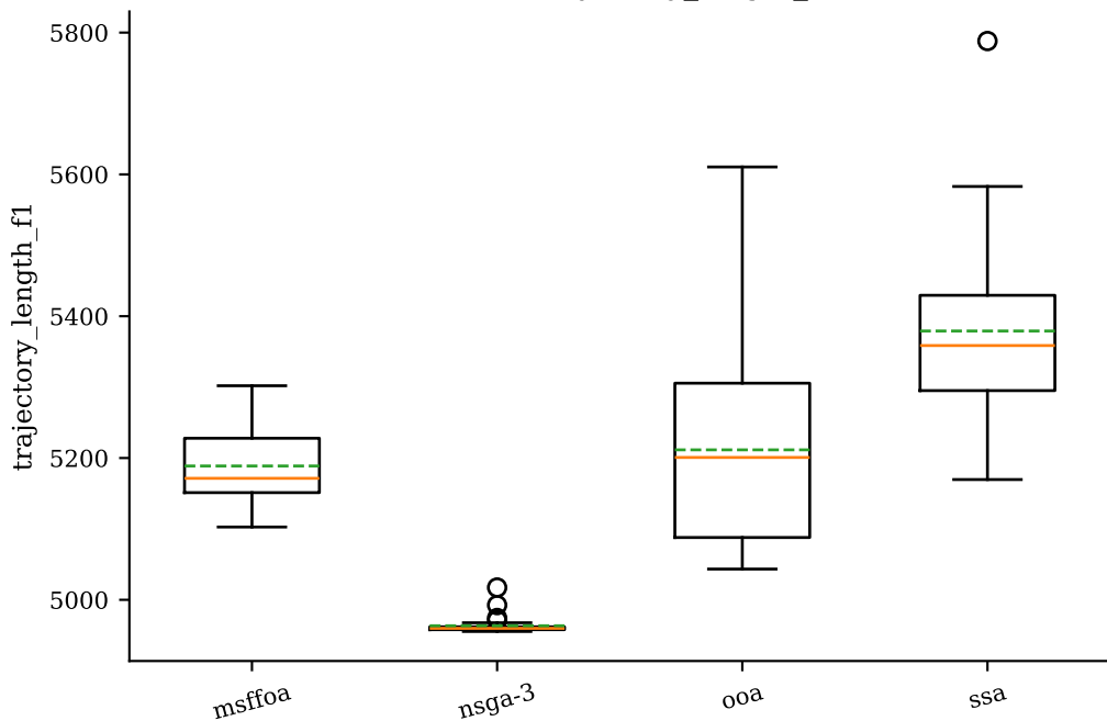
urban — trajectory_length_f1
