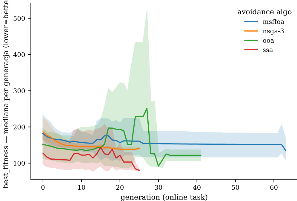
forest — Online optimizer convergence (§3.1.3.2 Krzywa optymalizacji)
