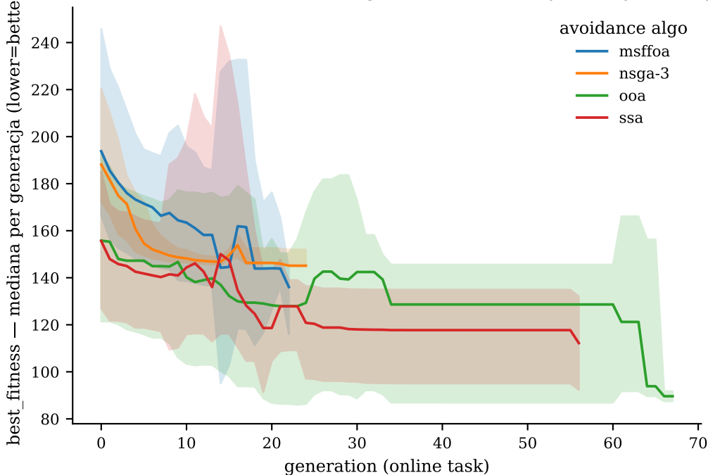
urban — Online optimizer convergence (§3.1.3.2 Krzywa optymalizacji)
