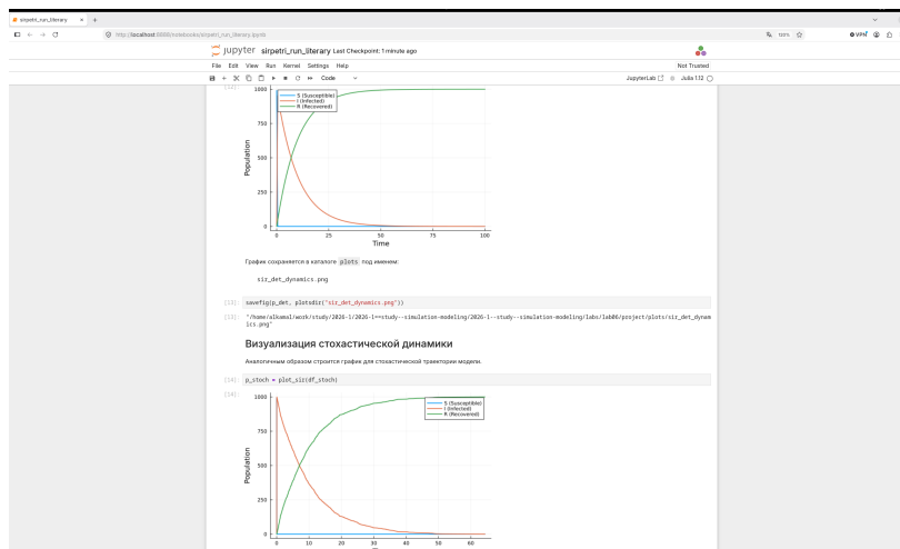
Рисунок 2.5: Детерминированная и стохастическая динамика модели SIR в Jupyter Notebook
