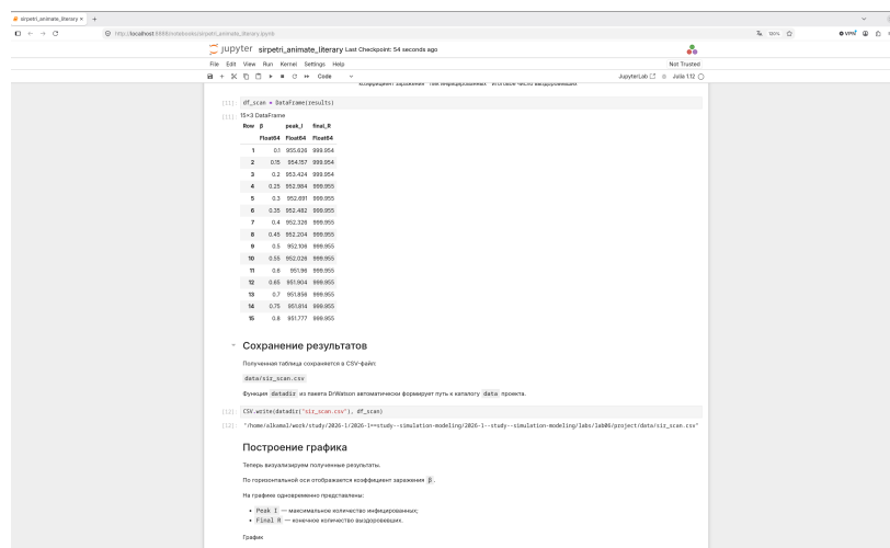
Рисунок 2.11: Таблица результатов и подготовка визуализации параметров модели SIR в Jupyter Notebook
