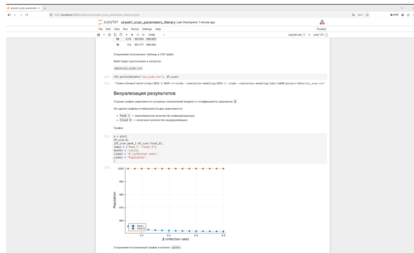
Рисунок 2.8: Зависимость показателей модели SIR от коэффициента заражения \beta
