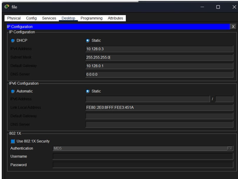
Рисунок 13: Настройка IP-адресации на сервере File
