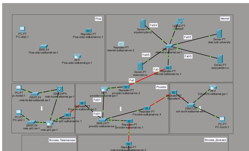
Рисунок 2.1: Топология сети Университета г. Пиза в логической рабочей области
