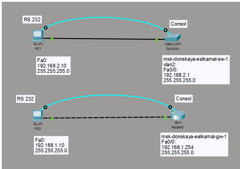
Рисунок 1: Топология сети с маршрутизатором, коммутатором и двумя ПК
