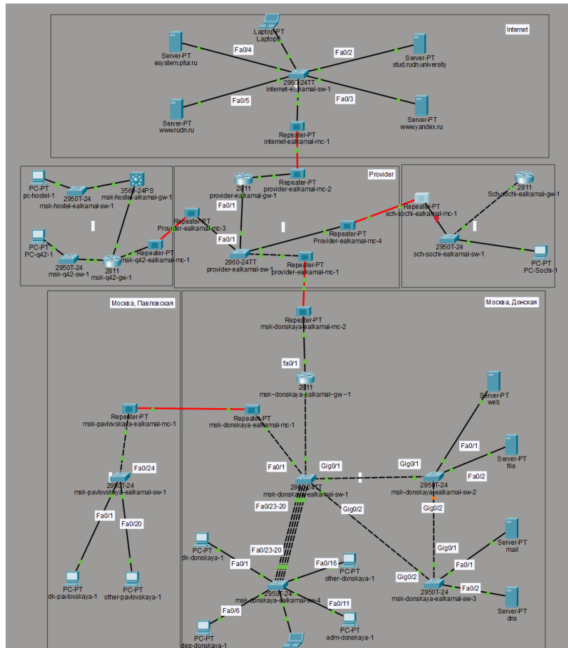
Рисунок 2.17: Итоговая топология сети после настройки
