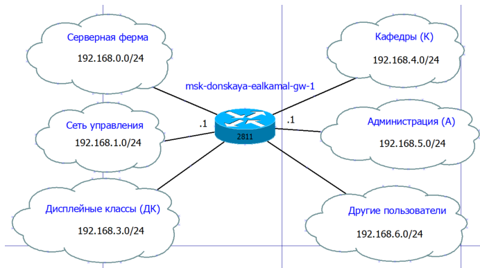
Рисунок 15: Повтор схемы L3 (сетевого уровень) в графическом редакторе Dia для сети 192.168.0.0/16
