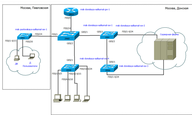
Рисунок 1: Повтор схемы L1 (физический уровень) в графическом редакторе Dia
