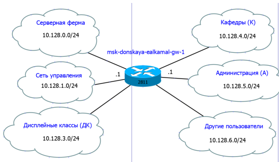
Рисунок 3: Повтор схемы L3 (сетевой уровень) в графическом редакторе Dia
