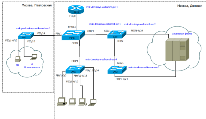
Рисунок 13: Повтор схемы L1 (физический уровень) в графическом редакторе Dia для сети 192.168.0.0/16
