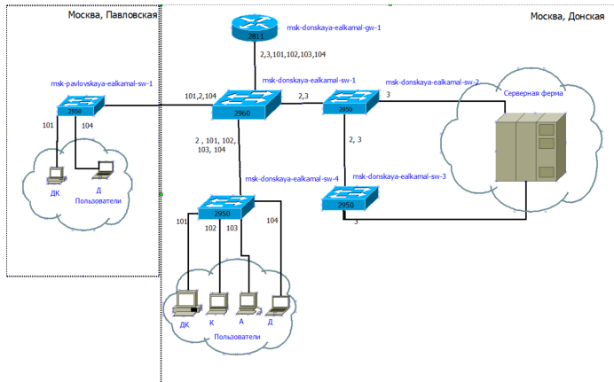
Рисунок 14: Повтор схемы L2 (канальный уровень) в графическом редакторе Dia для сети 192.168.0.0/16
