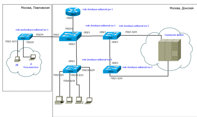
Рисунок 7: Повтор схемы L1 (физический уровень) в графическом редакторе Dia для сети 172.16.0.0/12
