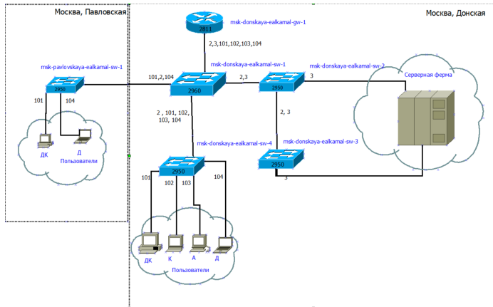
Рисунок 8: Повтор схемы L2 (канальный уровень) в графическом редакторе Dia для сети 172.16.0.0/12
