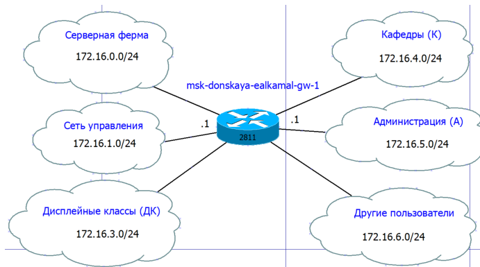
Рисунок 9: Повтор схемы L3 (сетевой уровень) в графическом редакторе Dia для сети 172.16.0.0/12
