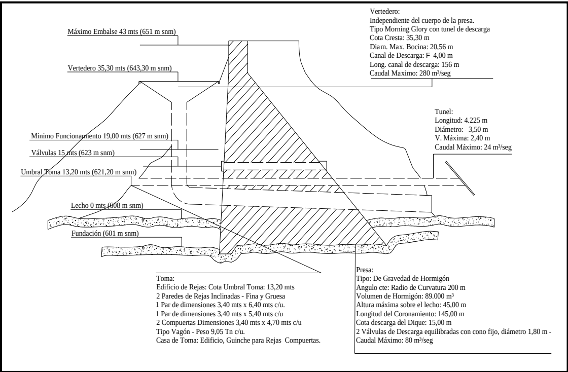
Ilustración 6: Corte esquemático del Dique San Roque
