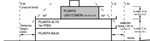
Ejemplo Alzada transversal a la calle Zona R Salientes de la L.E.
