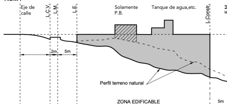
Ejemplo Alzada transversal a la calle RSM1
