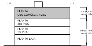
Ejemplo Alzada frente sobre calle C2
