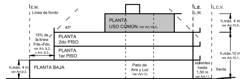
Ejemplo Alzada transversal a la calle AC2 Lote en esquina con salientes de la L.E.
