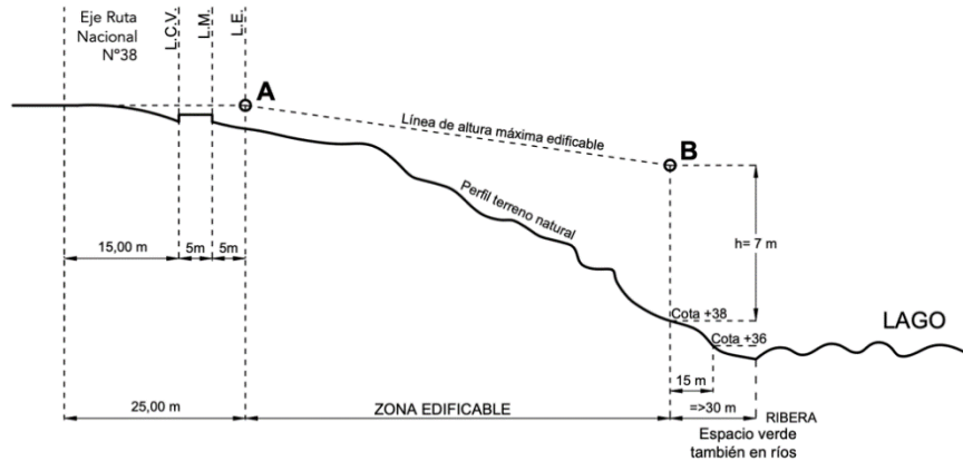
Ejemplo Alzada transversal Bv. Sarmiento - Ruta Nacional 38 R2
