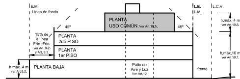
Ejemplo Alzada transversal a la calle AC2 Lote en esquina
