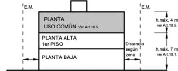
Ejemplo alzada frente sobre calle Zona R
