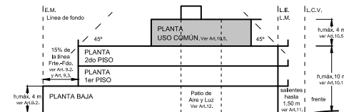
Ejemplo Alzada transversal a la calle C2 Salientes de la L.E.
