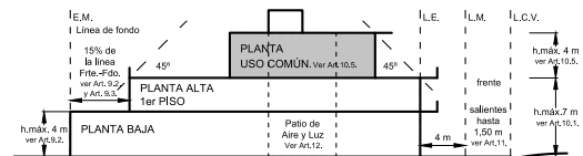
Ejemplo Alzada transversal a la calle AC1 Salientes de la L.E.
