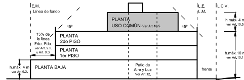
Ejemplo Alzada transversal a la calle C2
