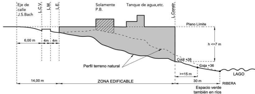
Ejemplo Alzada transversal a la calle J.S. Bach R2
