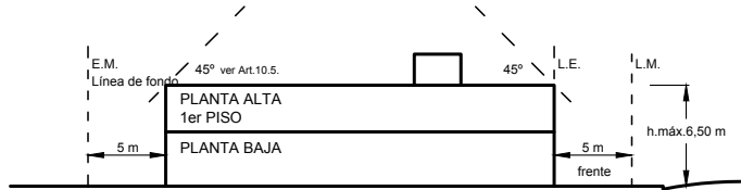
Ejemplo Alzada transversal a la calle RSM2
