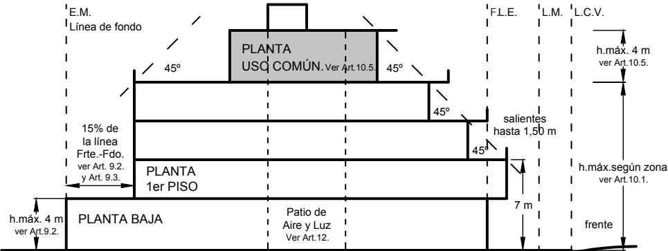
Ejemplo alzada transversal a la calle Salientes de la L.E. de cuerpos edilicios solamente en los casos encuadrados en el Art.5.2. Ensanche de calle.
