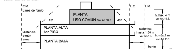
Ejemplo Alzada transversal a la calle Zona R Salientes de la L.E.
