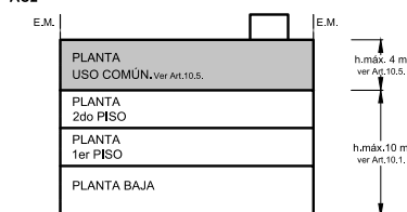
Ejemplo Alzada frente sobre calle AC2
