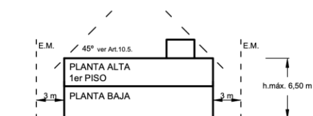
Ejemplo alzada frente sobre calle RSM2
