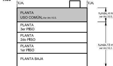
Ejemplo Alzada frente sobre calle AC3
