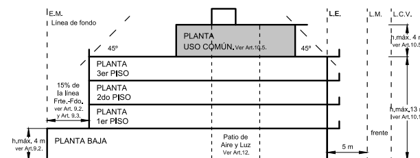
Ejemplo Alzada transversal a la calle C1 T1 Salientes de la L.E.
