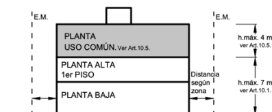
Ejemplo alzada frente sobre calle Zona R
