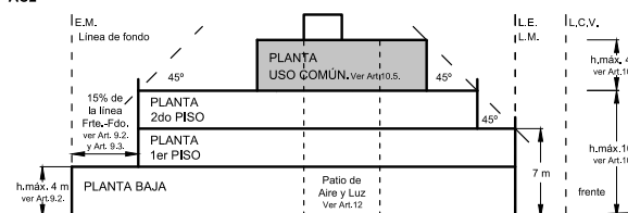
Ejemplo Alzada transversal a la calle AC2
