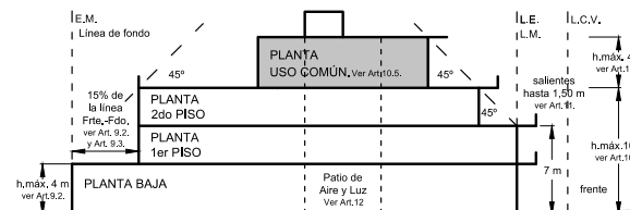
Ejemplo alzada transversal a la calle AC2 Salientes de la L.E.
