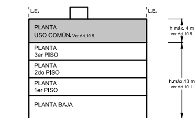
Ejemplo Alzada frente sobre calle C1 T2
