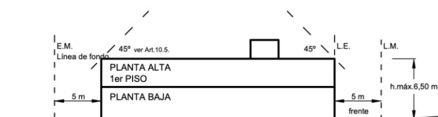
Ejemplo Alzada transversal a la calle RSM2
