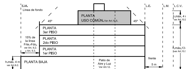
Ejemplo Alzada transversal a la calle C1 T1 Salientes de la L.E.
