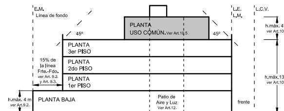
Ejemplo Alzada transversal a la calle
