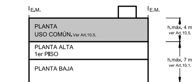
Ejemplo Alzada frente sobre calle AC1
