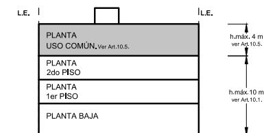
Ejemplo Alzada frente sobre calle C2
