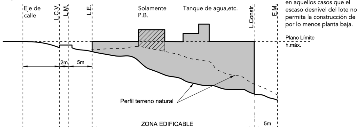
Ejemplo Alzada transversal a la calle RSM1
