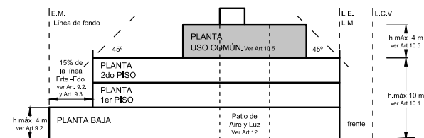
Ejemplo Alzada transversal a la calle C2
