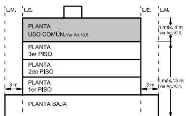
Ejemplo Alzada frente sobre calle C1 T1
