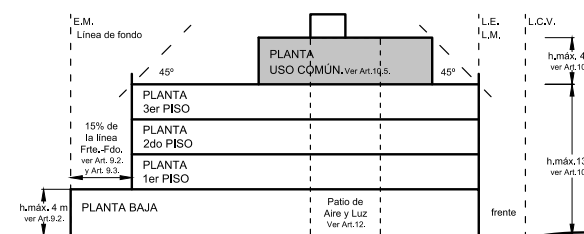
Ejemplo Alzada transversal a la calle C1 T2 Salientes de la L.E.
