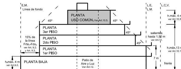
Ejemplo alzada transversal a la calle AC3 Salientes de la L.E.
