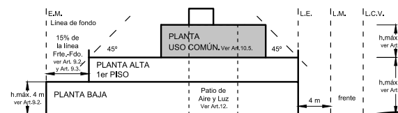
Ejemplo Alzada transversal a la calle AC1 Salientes de la L.E.
