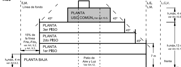
Ejemplo Alzada transversal a la calle AC3
