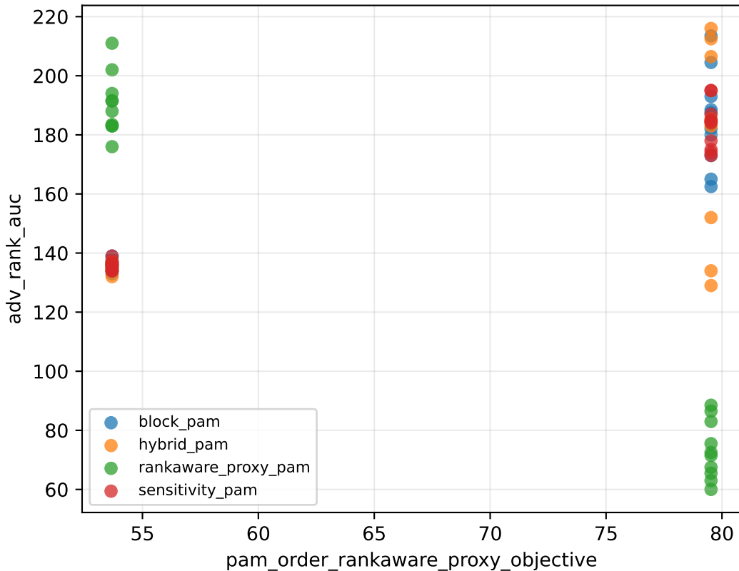
Static proxy vs actual rank-AUC
