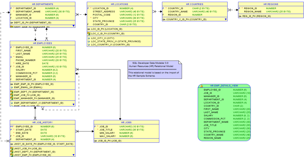
Figure 4: Schéma logique relationnel HR
