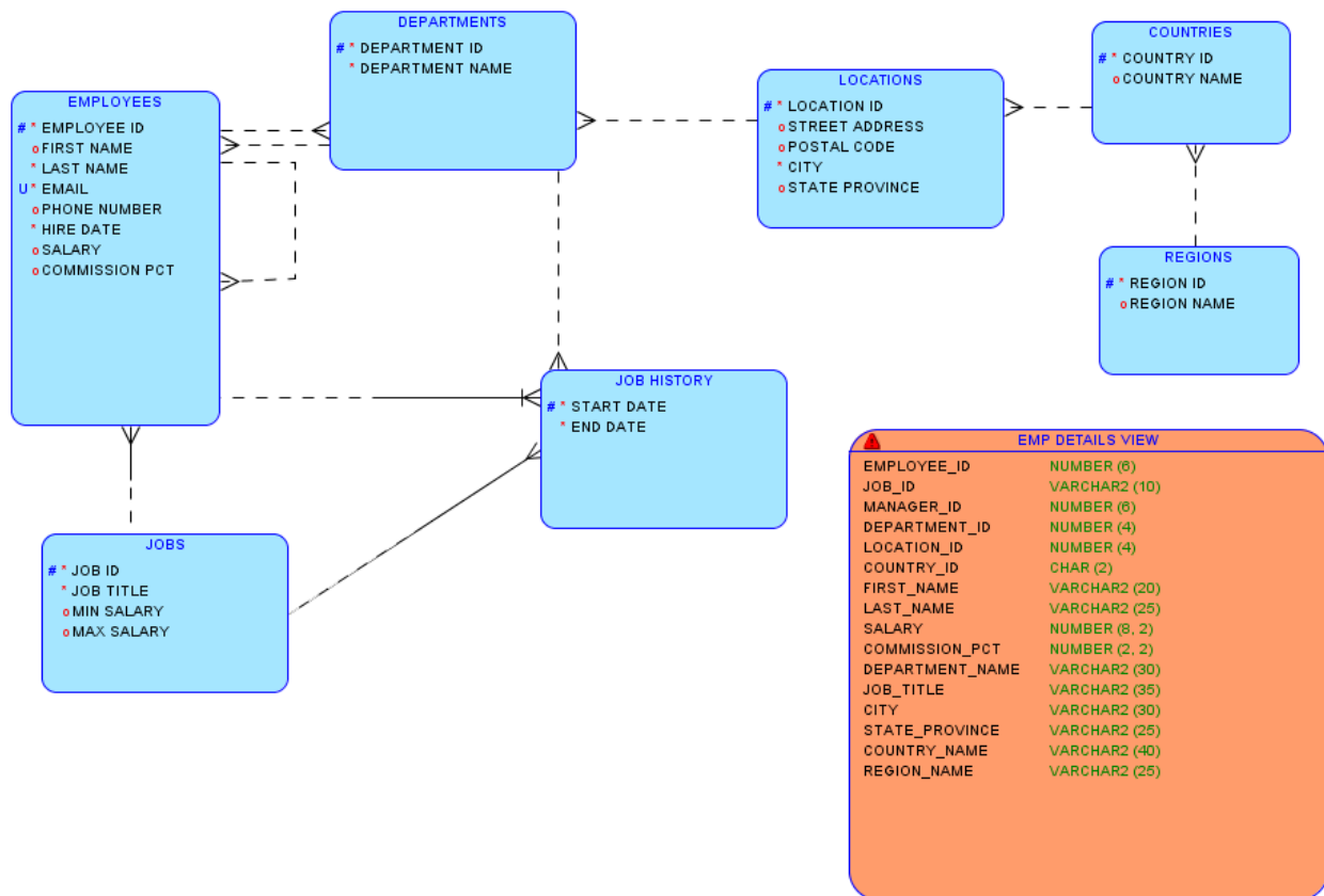
Figure 3 : Schéma conceptuel HR
