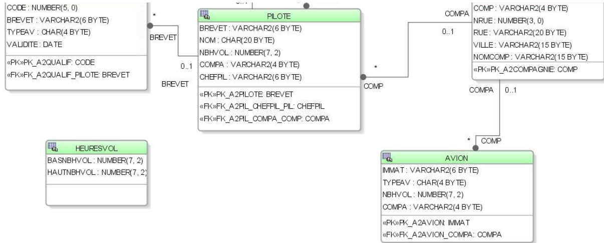
Figure 2 : Schéma conceptuel PILOTE
