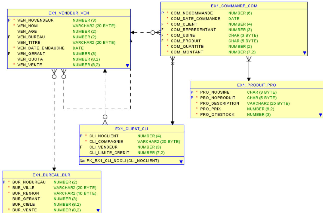
Figure 1: Schéma logique relationnel EX1
