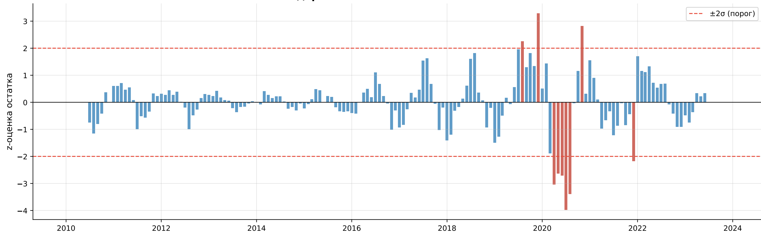
Стандартизованная остаточная компонента
